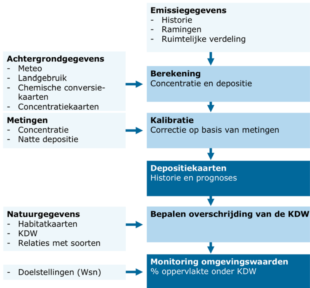
Figuur 3.1 Schematische weergave van de gehanteerde methode om de stikstofdepositie en de overschrijding van de kritische depositiewaarden te berekenen.
