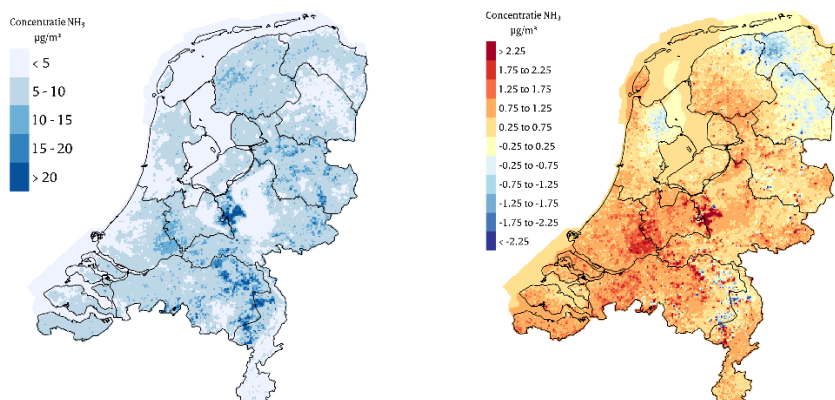
Figuur B.14 Grootschalige \text{NH}_3 -concentratie in 2025 (links) en het verschil tussen 2024 en 2025 (rechts), beide in \mu\text{g}/\text{m}^3 .
