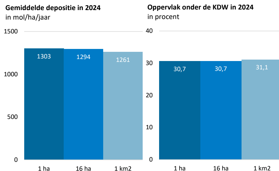
Figuur B.1 Effect van resolutie van de kaarten op de gemiddelde depositie en het percentage niet-overbelast areaal stikstofgevoelige natuur in Natura 2000-gebieden in 2024 (op basis van gemiddelde weersomstandigheden).
