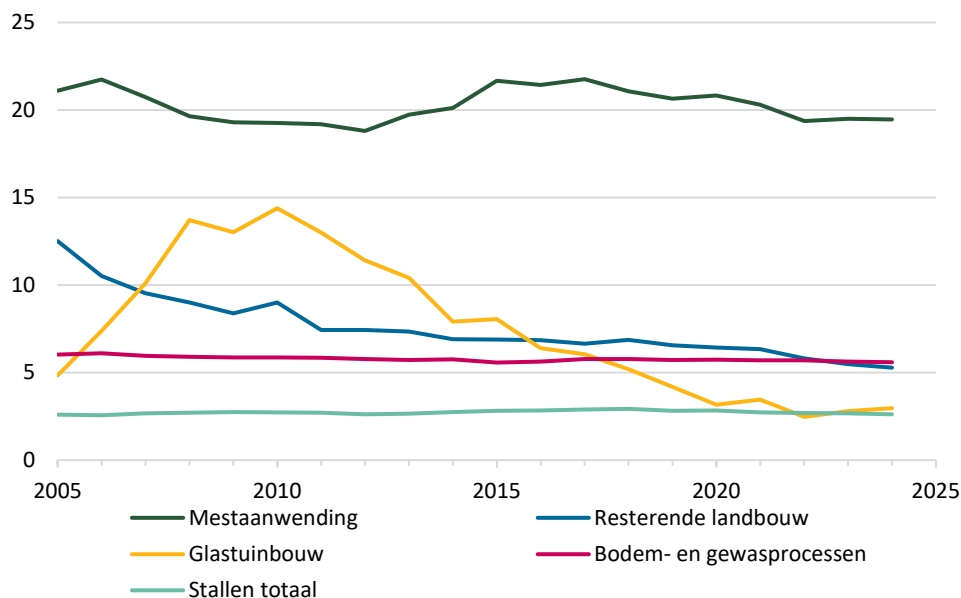
Figuur 4.4 Ontwikkeling van de emissies van stikstofoxiden door de Nederlandse landbouwsector in de periode 2005-2024.
