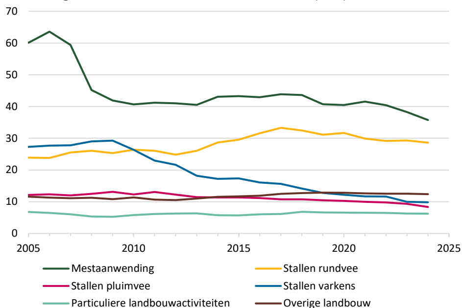
Figuur 4.3 Ontwikkeling van de ammoniakemissies door de Nederlandse landbouwsector in de periode 2005-2024.
