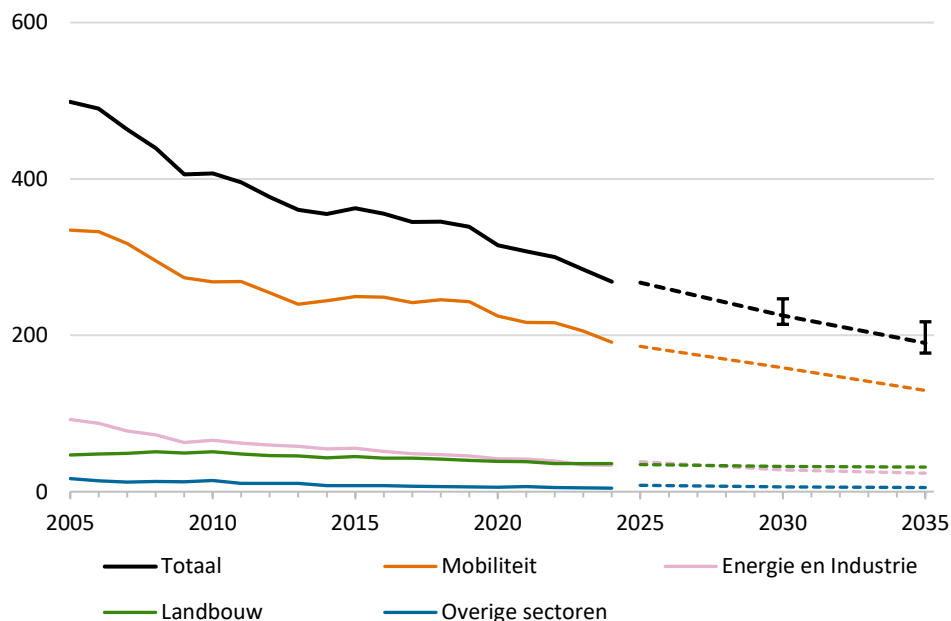
Figuur 4.2 Ontwikkeling van de Nederlandse emissies van stikstofoxiden naar sector.
