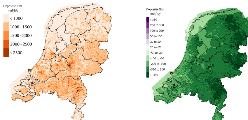
Figuur B.15 Grootschalige stikstofdepositie in 2025 (links) en het verschil tussen 2024 en 2025 (rechts), beide in mol per hectare per jaar.
