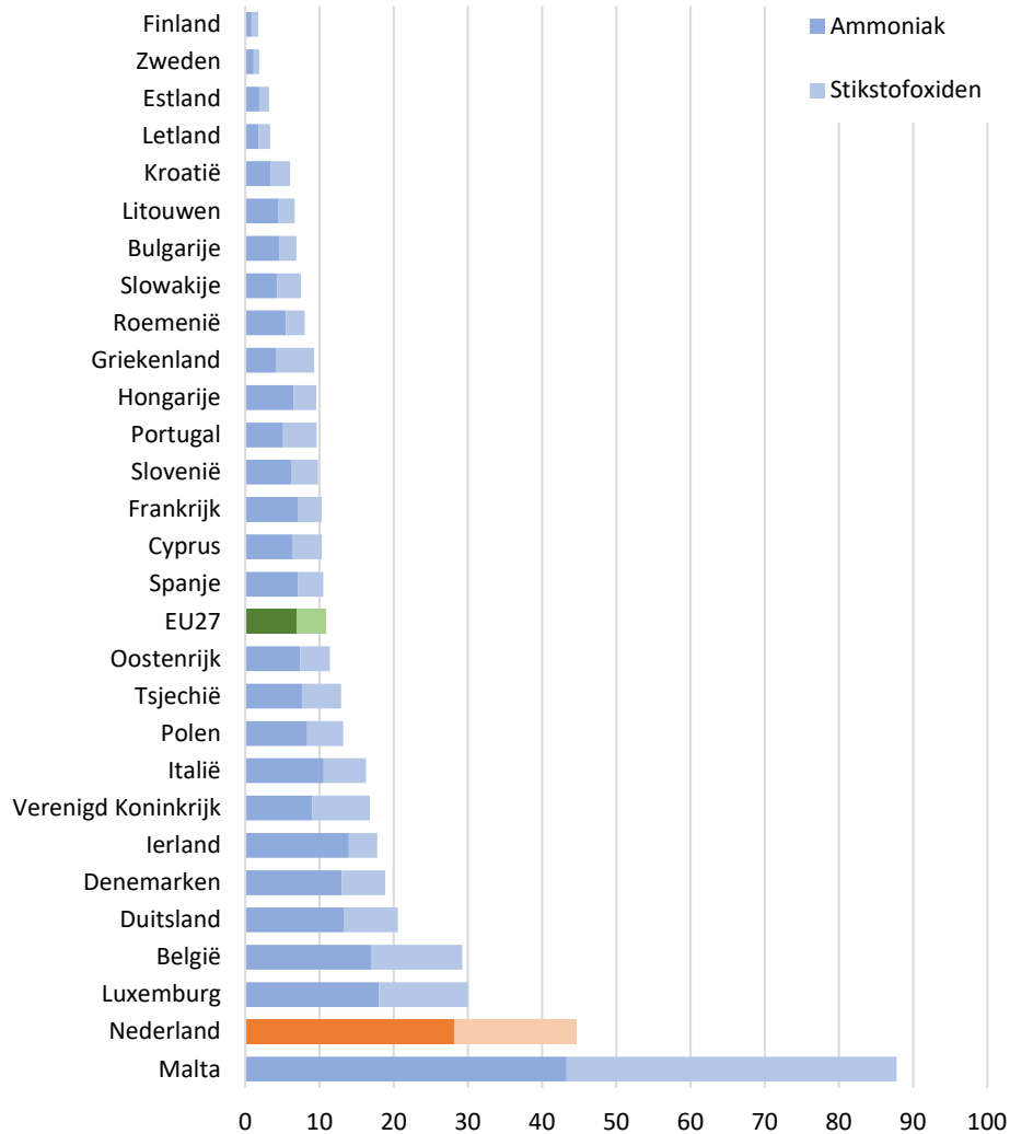
Figuur 4.6 Stikstofemissies in 2023 in kg N per hectare per jaar voor alle 27 EU-landen en het Verenigd Koninkrijk.
