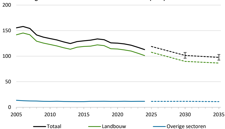
Figuur 4.1 Ontwikkeling van de Nederlandse ammoniakemissies naar sector.
