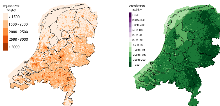
Figuur B.16 Grootschalige verzurende depositie in 2025 (links) en het verschil tussen 2024 en 2025 (rechts), beide in mol zuurequivalenten per hectare per jaar.
