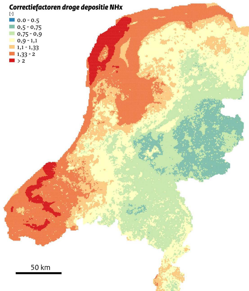
Figuur B.3 Correctiefactoren droge depositie \text{NH}_x , gebaseerd op het vijfjarig verschil tussen modelresultaten en metingen voor de jaren 2020 t/m 2024.
