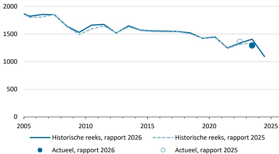
Figuur B.9 Ontwikkeling van overschrijding van de kritische depositiewaarde: de historische reeks uit rapportage 2025 (lichtblauwe lijn), de historische reeks uit rapportage 2026 (donkerblauwe lijn), de actuele depositie (2023) uit rapportage 2025 (open cirkel) en de actuele depositie (2024) uit rapportage 2026 (gesloten cirkel). Door de gehanteerde methode kunnen de lijnen onderling worden vergeleken en de cirkels onderling worden vergeleken.
