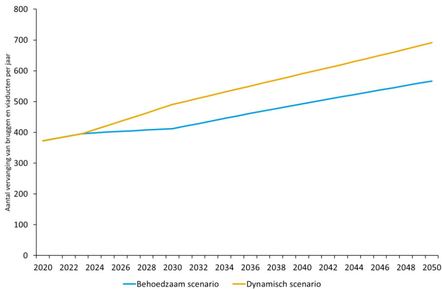
Afbeelding 4.15 Prognose vervanging aantal bruggen en viaducten (exclusief hout) alle publieke opdrachtgevers, 2020-2050
