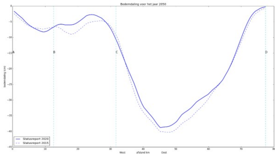
Figuur 29; Doorsnede van de bodemdalingssom in Friesland en Groningen. Vergelijking van de gemodelleerde bodemdaling in 2050 volgens het Statusrapport 2015 en 2020.
