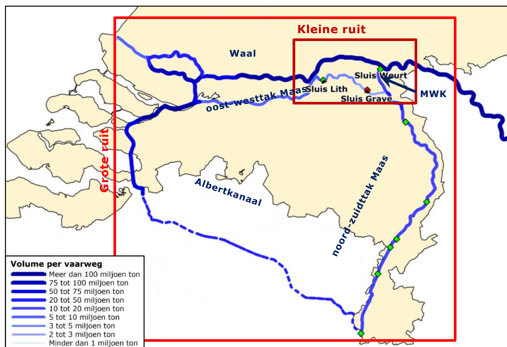
Figuur 1: Overzicht van het vaarwegennetwerk en de sluizen, inclusief volumes in het jaar 2019 (bron: Panteia, gebaseerd op BIVAS) – MWK = Maaswaalkanaal
