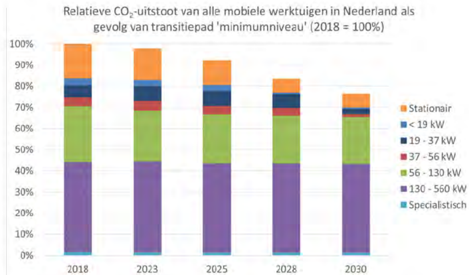
Figuur 3: Potentiële reductie van CO 2 -emissies in 2030 ten opzichte van 2018 als gevolg van het minimumniveau.
