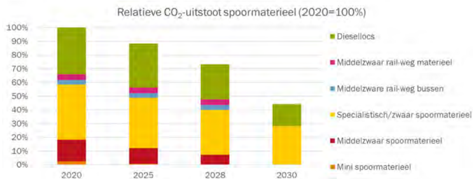
Figuur 7: CO 2 -reductie voor 2025, 2028 en 2030 ten opzichte van 2020 van spoor specialistisch materieel ten gevolge van het ambitieuze niveau.
