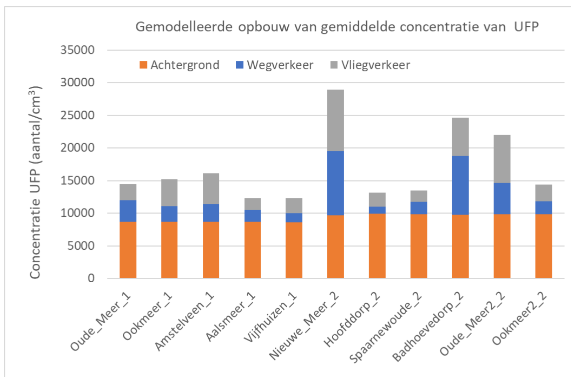
Figuur 4 Indicatie van de concentratieopbouw van ultrafijn stof op de meetlocaties, bepaald met het rekenmodel. _1 betreft de 1e meetperiode (augustus 2017-januari 2018), _2 de 2e meetperiode (maart-augustus 2018).
