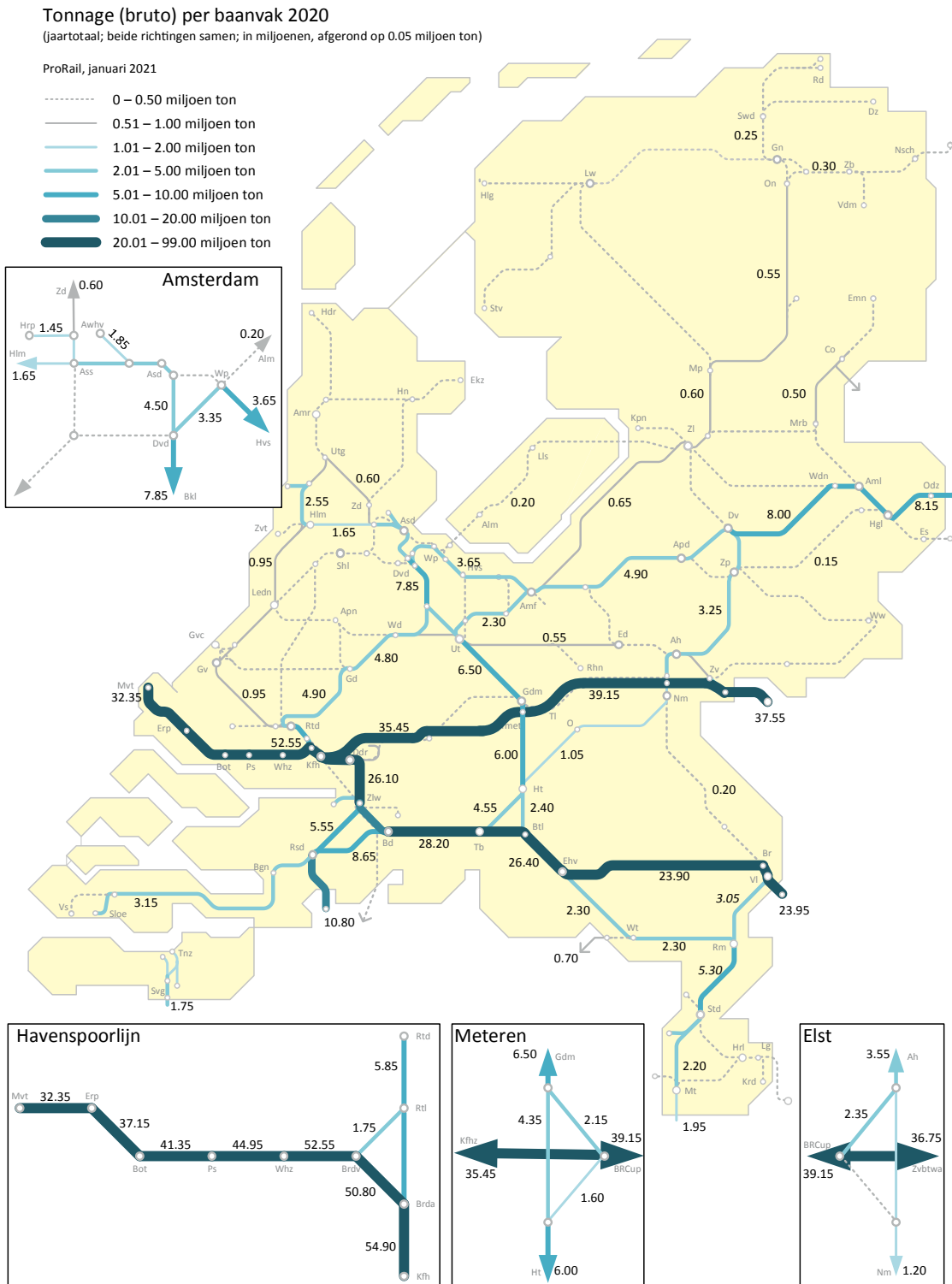
Figuur 3.5: tonnage (bruto) per baanvak in 2020
