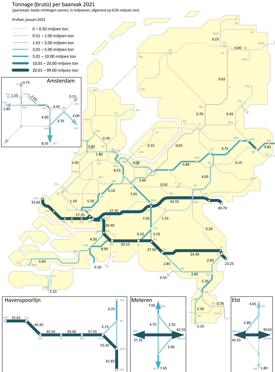
Figuur 3.6: tonnage (bruto) per baanvak in 2021
