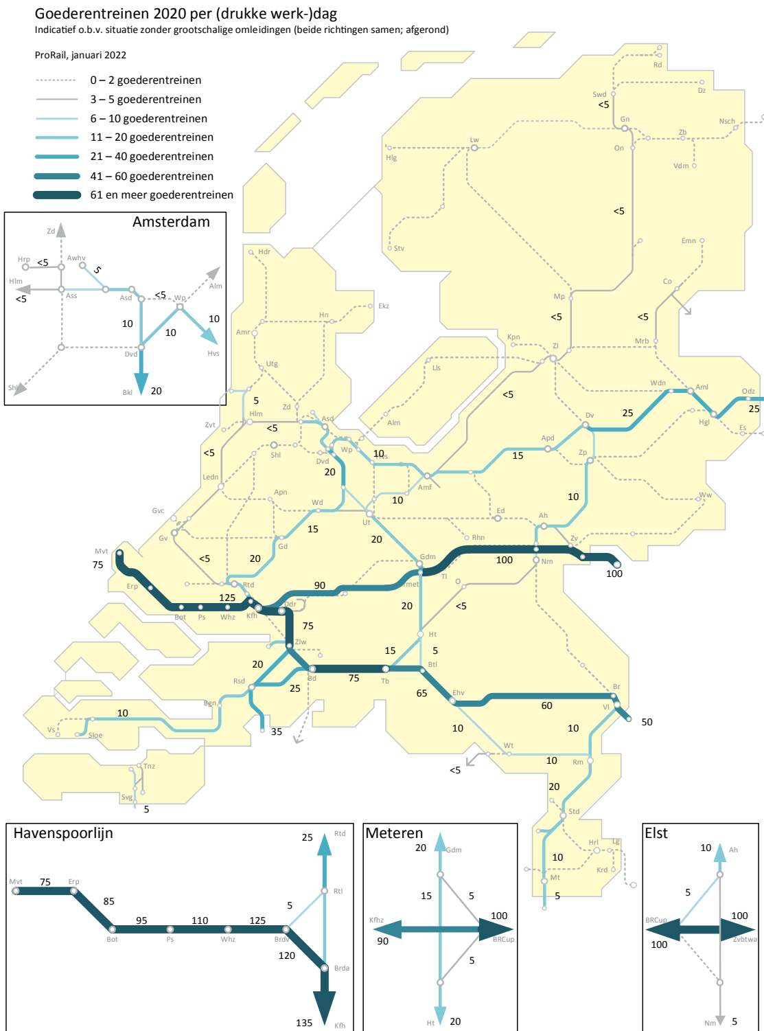
Figuur BI.1: aantal goederentreinen werk (drukke) werkdag in 2020 in situatie zonder omleidingen vanwege de bouw van het 3 e spoor Zevenaar – Oberhausen
