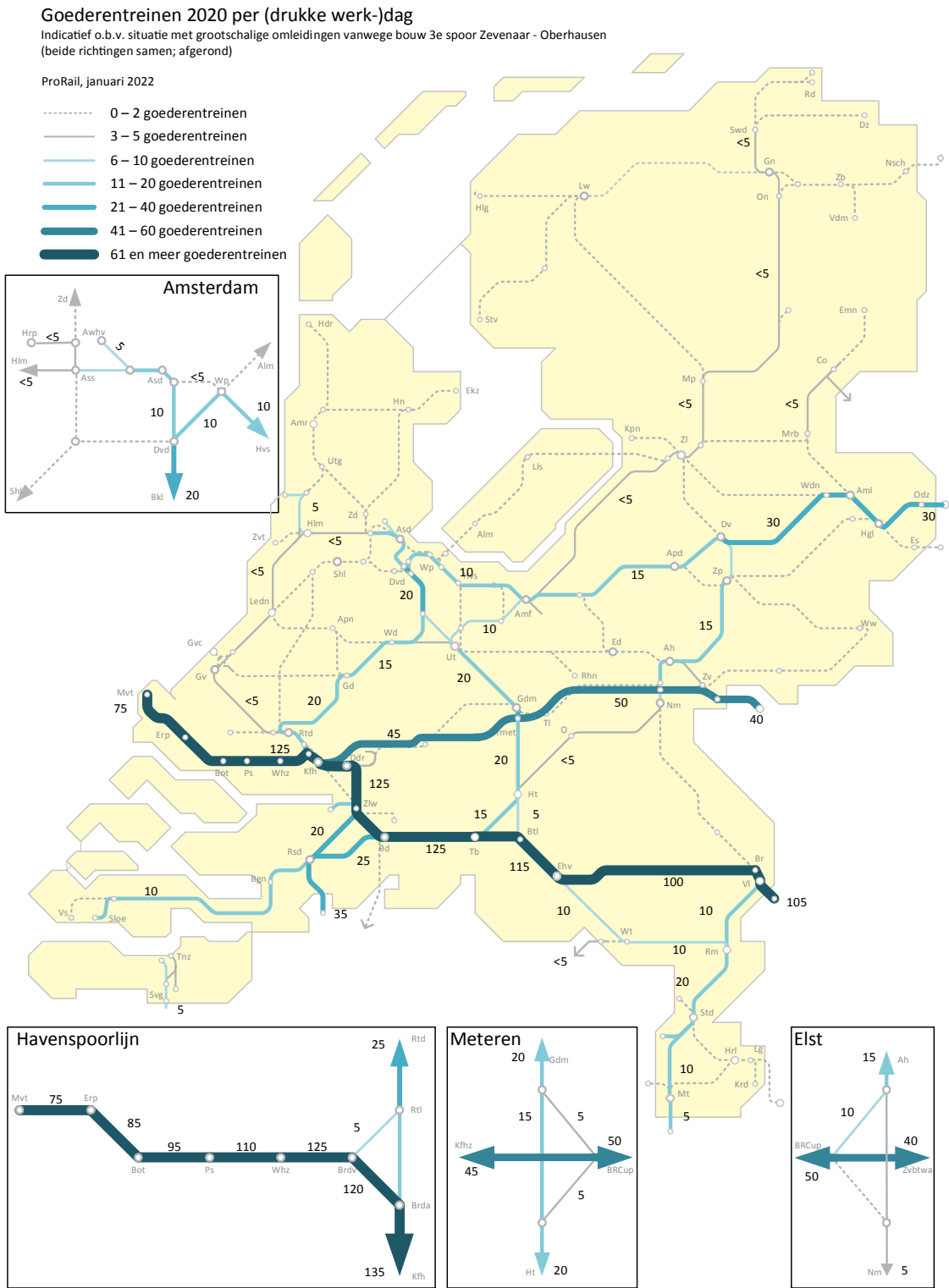
Figuur BI.2: aantal goederentreinen werk (drukke) werkdag in 2020 in situatie met omleidingen vanwege de bouw van het 3 e spoor Zevenaar – Oberhausen
