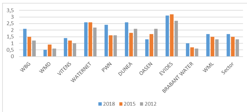
Prestatievergelijking 2019 Figuur 4.5 NIRG per kilometer leiding (m³/km/dag) 2012-2018
