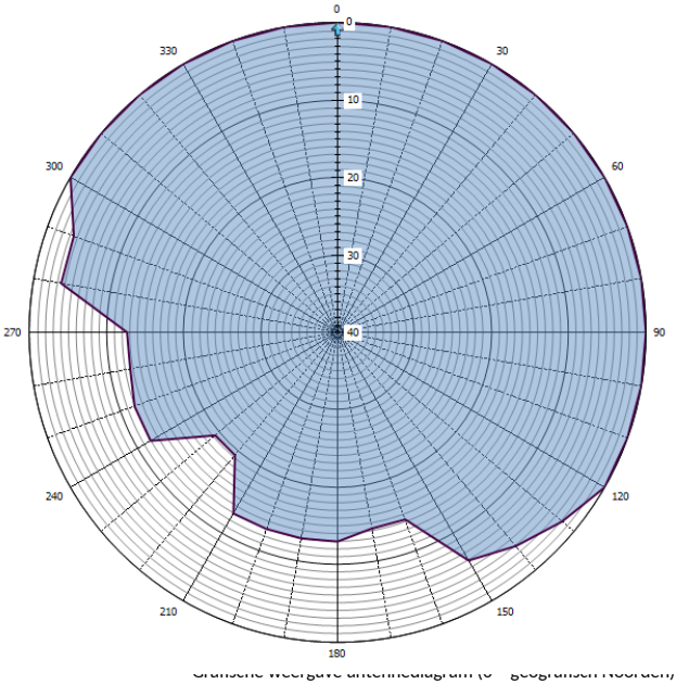
Grens van toegewezen antennegebied (niet begrensd gebied)
