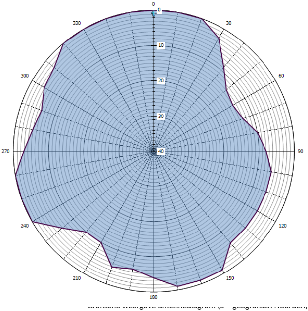
Statische draagbereiksberekening (gegevens m.b.t. antennesysteem)
