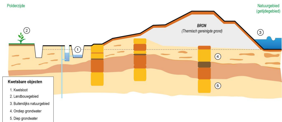
Figuur 2.3 Schematische weergave van de zeedijk, aanwezigheid van thermisch gereinigde grond (TGG, kwetsbare objecten en bodemopbouw: geel = zand, rood-bruin = klei en donkerbruin = veen. De bodemopbouw ter plaatse van de intensere kleuren is afgeleid op basis van uitgevoerde boringen
