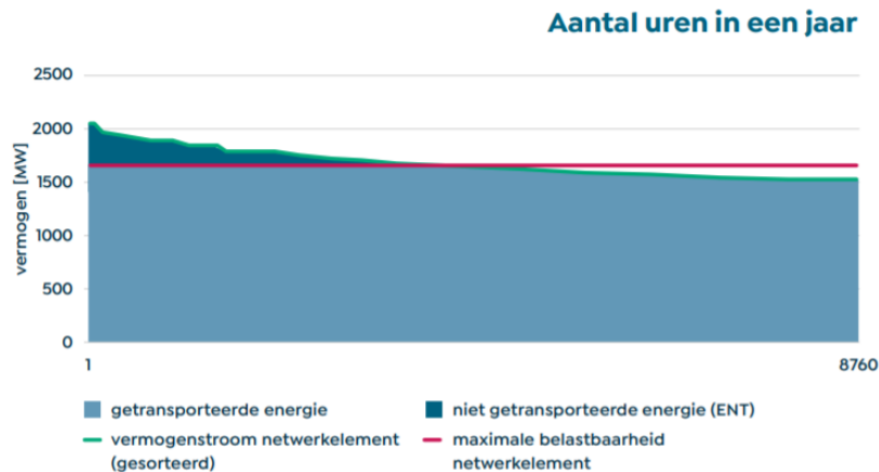
Figuur 18: Schematische weergave ENT
