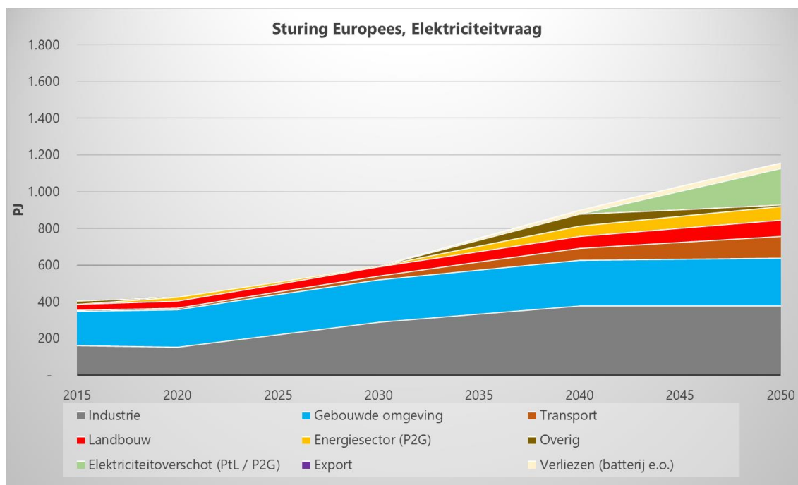
Figuur 75. Ontwikkeling elektriciteitsvraag 2015-2050 scenario Europees.
