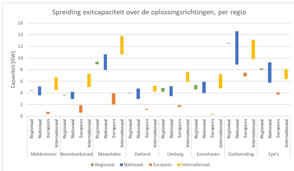
Figuur 52: Spreiding exitcapaciteit gezien over alle oplossingsrichtingen per regio voor het voorziene waterstofnetwerk.
