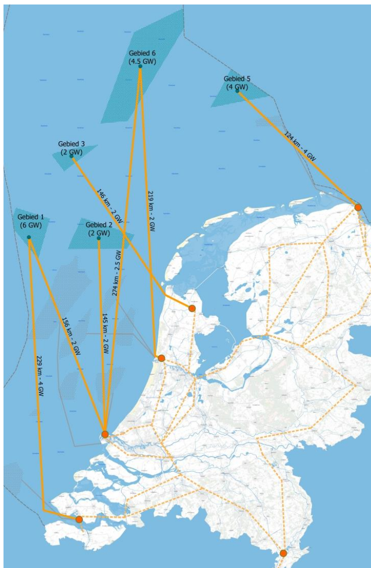
Figuur 7: Voorbeeld aansluiting wind op zee naar aanlandingslocaties
