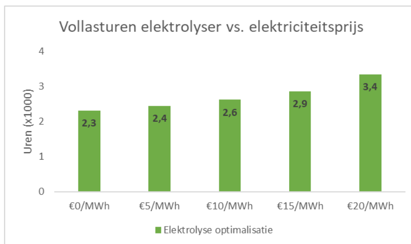
Figuur 58: Gevoeligheid elektrolyser vollasturen voor prijs overschotten elektriciteit
