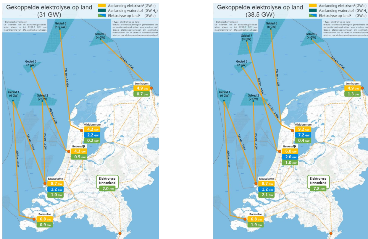
Figuur 27: Configuratie voor oplossingsrichting met elektrische ontsluiting op zee met gekoppelde elektrolyse op land.
