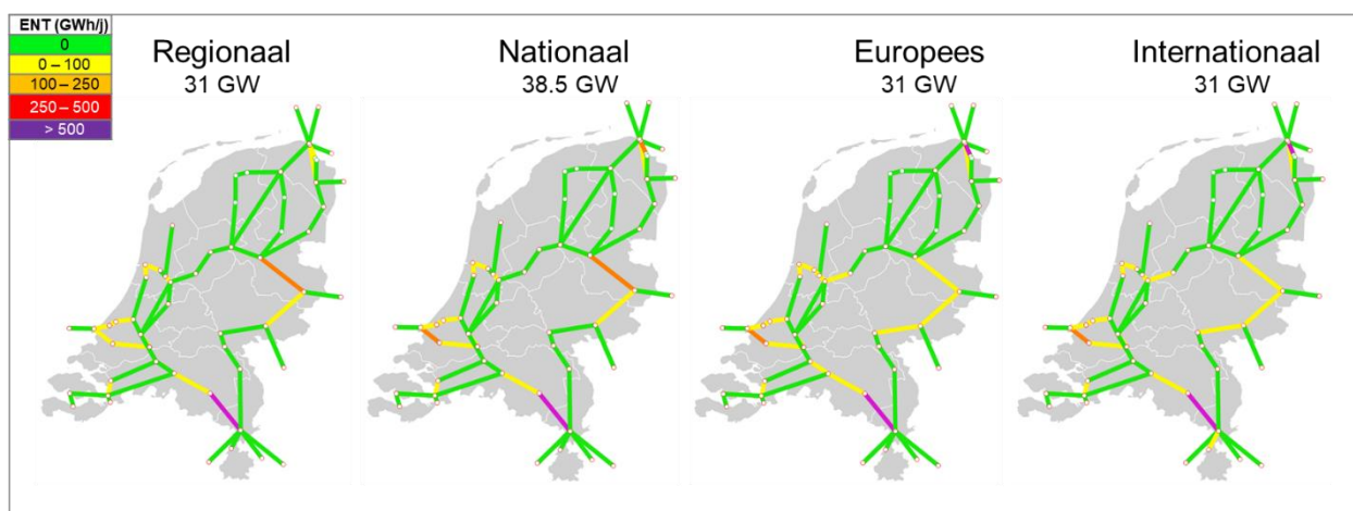
Figuur 48: Congestie elektriciteitsnet bij een volledig elektrische oplossingsrichting met elektrolyse ter preventie van congestie.
