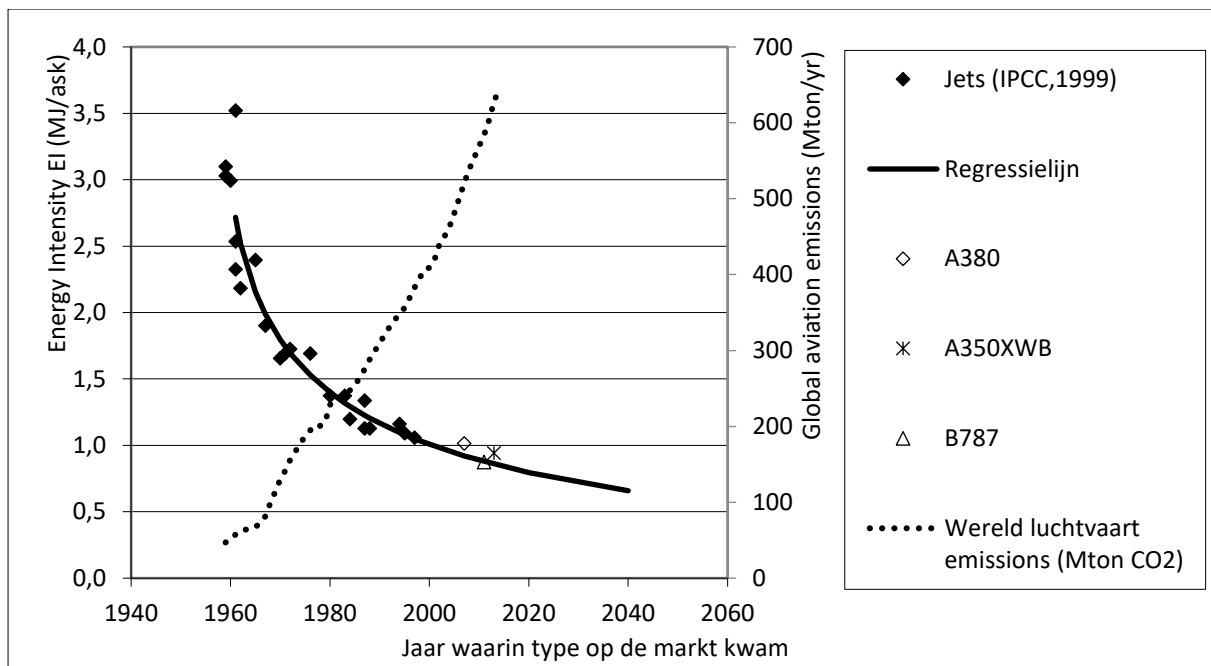
Figuur 8: Ontwikkeling van de brandstofefficiëntie van vliegtuigtypes in het verleden en met een projectie voor de toekomst (Peeters & Middel, 2007). De totale emissies zijn gebaseerd op Peeters (2017)
