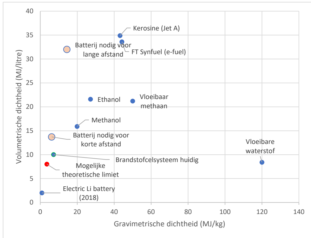
Figuur 9: Overzicht van de energiedichtheid met betrekking tot gewicht en volume voor kerosine, alternatieve brandstoffen en batterijen, brandstofcelsysteem huidige technologie op diverse studies.
