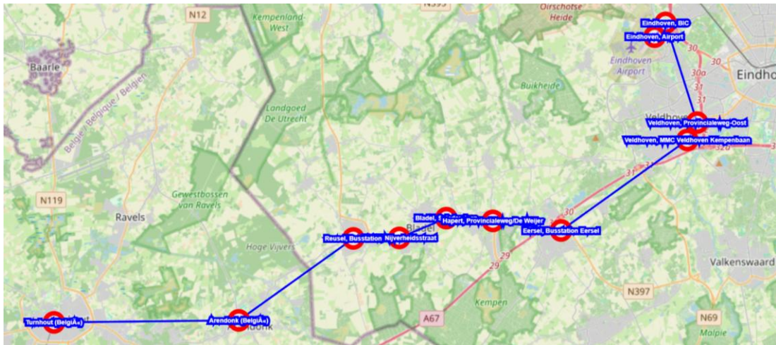
Figuur 5.4: onderzoeklijn Eindhoven - Turnhout
