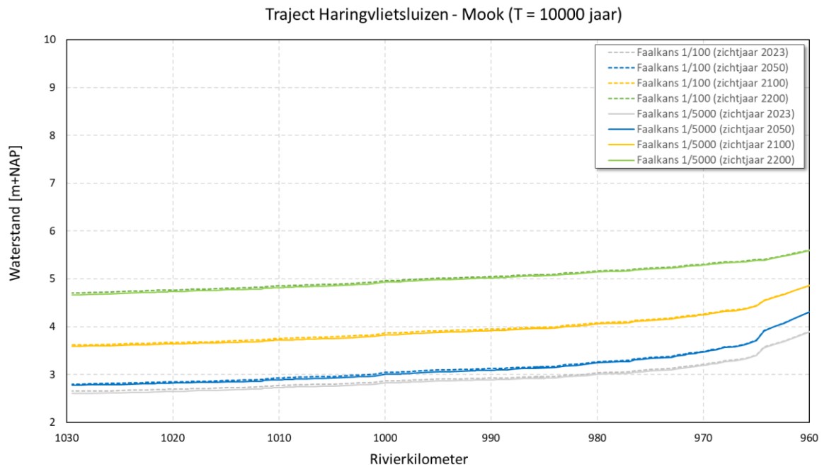
Figuur 5.5: Waterstand voor referentiesituatie met faalkans Maeslantkering 1/100 per sluitvraag (gestippelde lijn) en de variant met een tweede stormvloedkering met faalkans 1/5.000 per sluitvraag (doorgetrokken lijn) voor zichtjaren 2023 (grijs), 2050 (blauw), 2100 (geel) en 2200 (groen) – tracé Haringvlietsluizen tot Mook bij herhalingsstijd T = 10.000 jaar.
