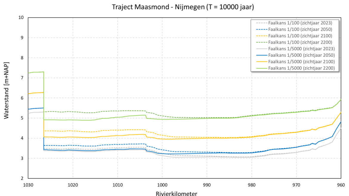
Figuur 5.3: Waterstand voor referentiesituatie met faalkans Maeslantkering 1/100 per sluitvraag (gestippelde lijn) en de variant met een tweede stormvloedkering met faalkans 1/5.000 per sluitvraag (doorgetrokken lijn) voor zichtjaren 2023 (grijs), 2050 (blauw), 2100 (geel) en 2200 (groen) – tracé Maasmond tot Nijmegen bij herhalingstijd T = 10.000 jaar.
