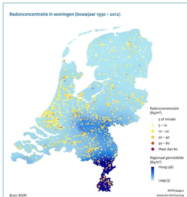
Figuur 4 Geografische weergave van de radonconcentratie in Nederlandse woningen 40 .
