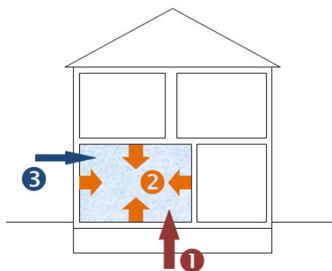
Figuur 2 Herkomst van radon in het binnenmilieu van woningen en gebouwen 14 .
