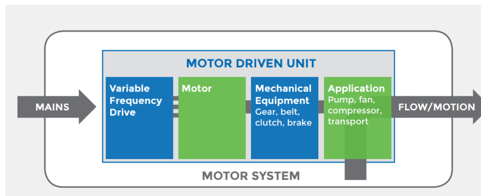
Figuur 5.9: schematische weergave motorgedreven systeem (U4E, 2017).
