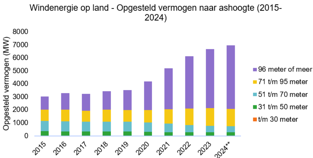
Figuur 5.5: Jaarlijks opgesteld vermogen wind op land, uitgesplitst naar ashoogte van de turbines. (CBS, 2025b).
