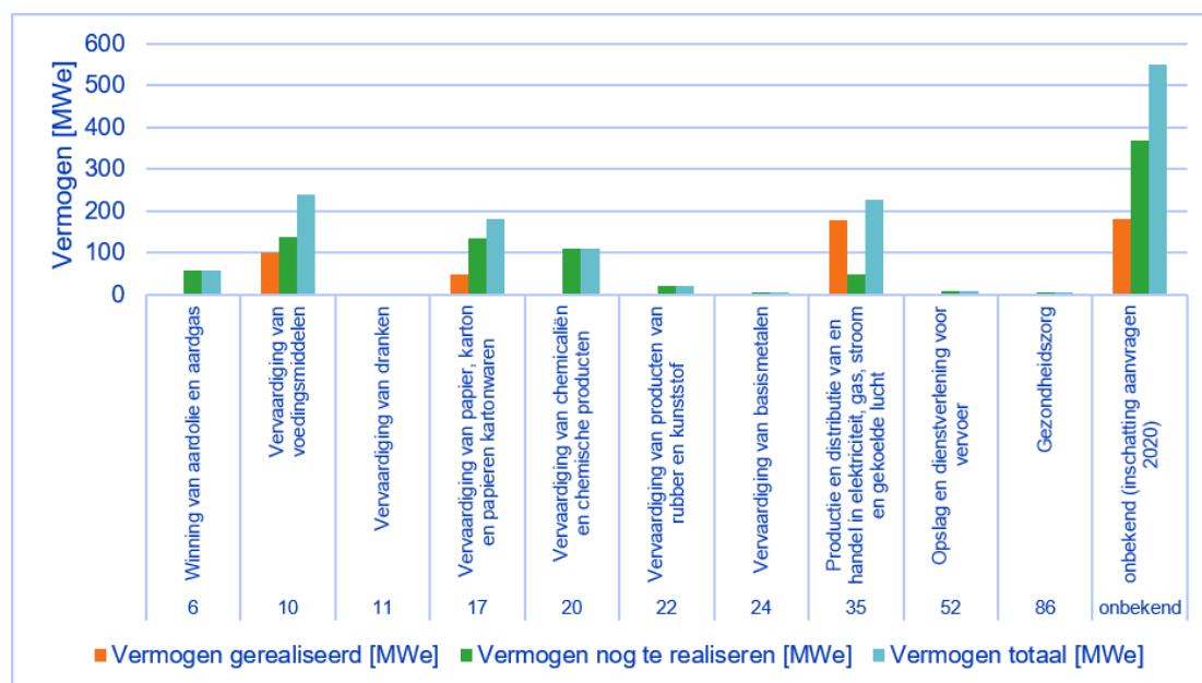
Figuur 4.5: SDE++ aanvragen e-boilers naar sector. Bewerking op (RVO, 2025).
