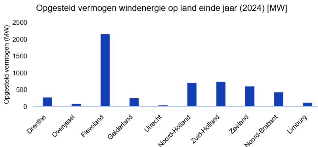
Figuur 5.6: Opgesteld vermogen windenergie op land eind 2024 (CBS, 2025c).
