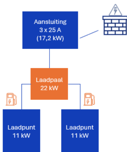
Figuur 4.9: Schematische weergave publieke laadpunten, laadpaal en de aansluiting.
