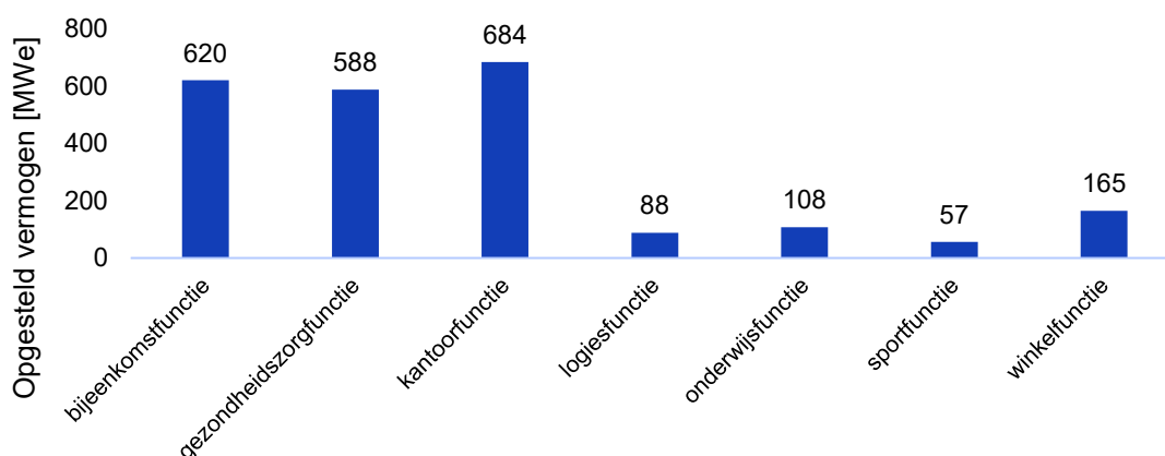
Figuur 4.3: Opgesteld vermogen warmtepompen per gebruiksfunctie in 2027.
