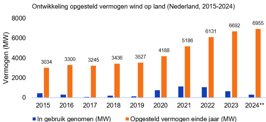
Figuur 4.11: Jaarlijks opgesteld vermogen en netto toename wind op land (CBS, 2025c).
