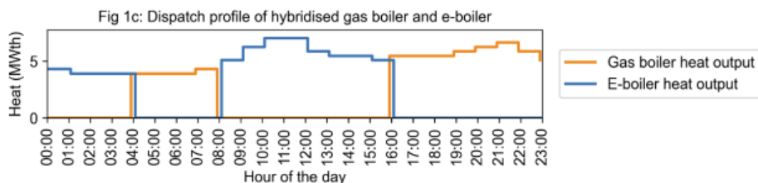
Figuur 4.6: Dispatch profile van hybride gasboiler en e-boiler toepassing (Oxenaar & Butler, 2026).
