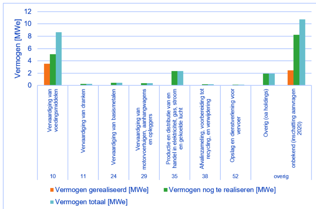
Figuur 4.8: Opgesteld vermogen naar aanvraag SDE++ subsidie industriële warmtepomp naar sector (RVO, 2025).
