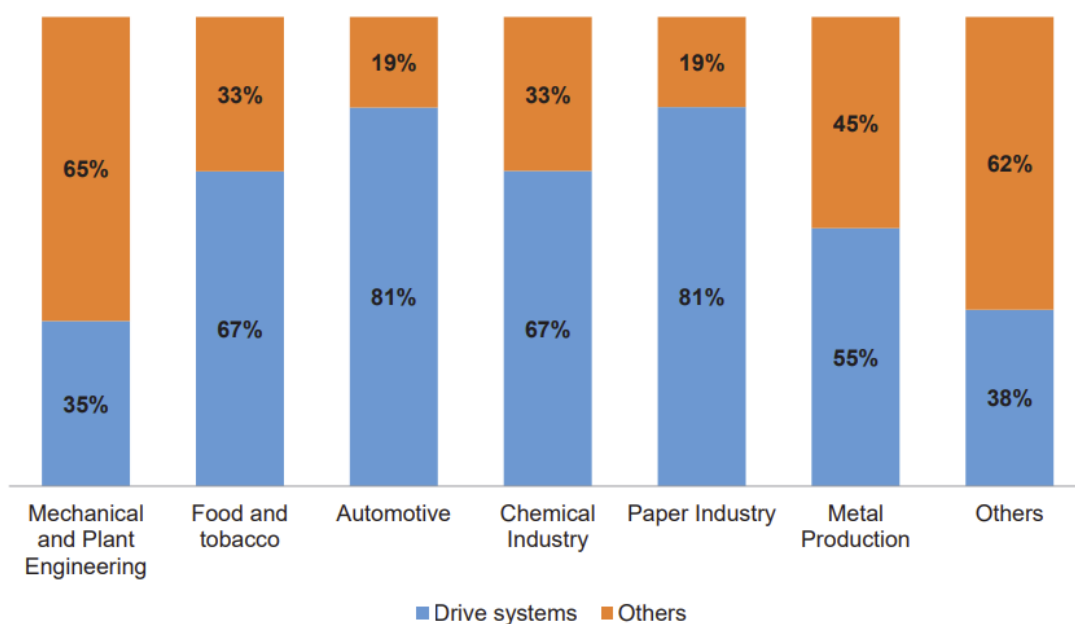
Figuur 5.8: Aandeel elektrische aandrijfsystemen in totaal elektriciteitsverbruik per sector in Duitsland (Javied, 2016).
