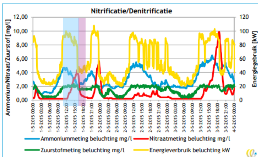
Figuur 4.2: Voorbeeld van fluctuerend energieverbruik van beluchting (gele lijn) ten opzichte van sturingsparameters (CE Delft, 2019)
