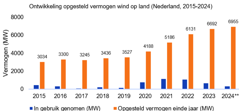
Figuur 5.4: Jaarlijks opgesteld vermogen en netto toename wind op land. (CBS, 2025c).
