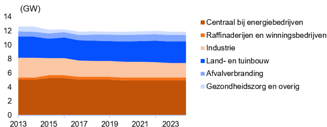
Figuur 4.12: Opgesteld warmtekrachtvermogen (Compendium voor de Leefomgeving, 2026).
