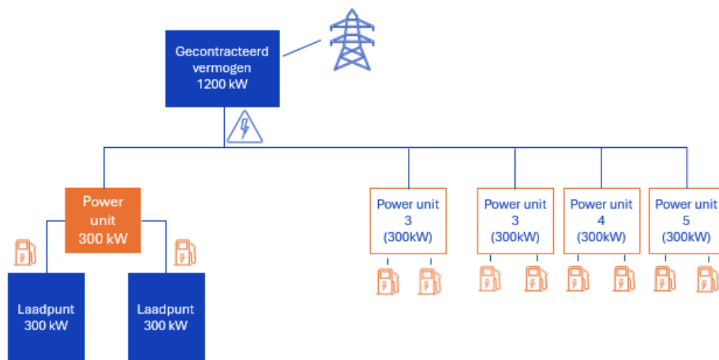
Figuur 4.10: Schematische weergave laadplein met laadpunten, power units en gecontracteerd vermogen op (bewerking op laadplein Shell (TNO, 2025c)).
