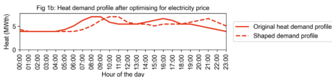
Figuur 4.7: Optimaliseren warmtevraag naar elektriciteitsprijs (Oxenaar & Butler, 2026).
