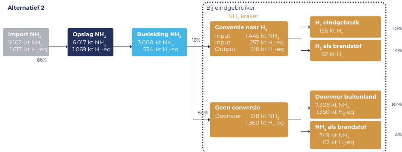
Figuur 4 Ketenelementen en totale volumes op jaarbasis in alternatief 2. De kleuren komen overeen met de legenda van figuur 2.
