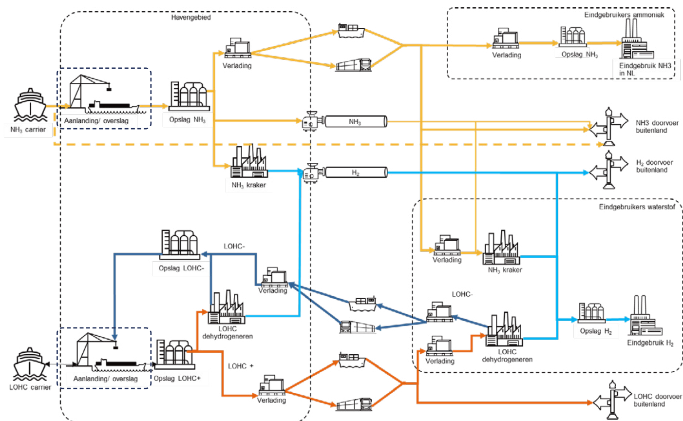
Figuur 26 Plaats van aanlanding/overslag in de ketens.
