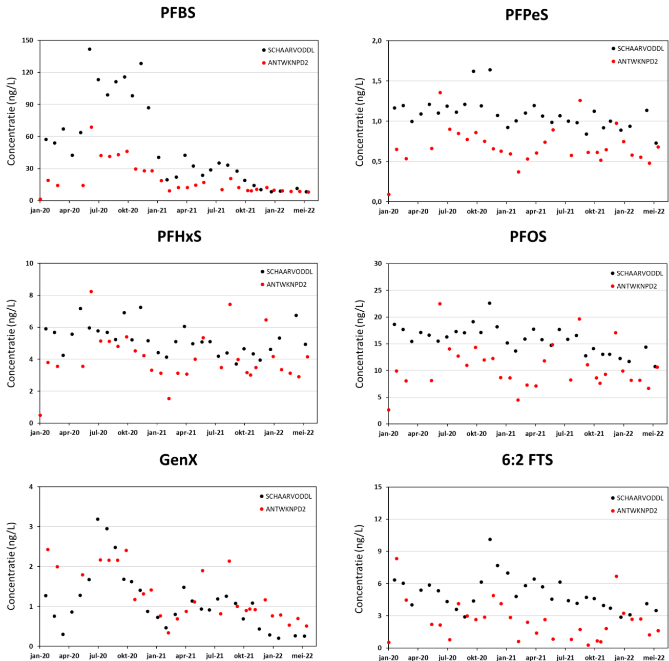
Figuur 13B: Resultaten van de maandelijkse concentratiemetingen in 2020-2022 van zes PFAS (PFBS, PFPeS, PFHxS, PFOS, GenX en 6:2 FTS) ) in het Antwerps Kanaalpand (ANTWKNPD2) en de Westerschelde (SCHAARVODDL).
