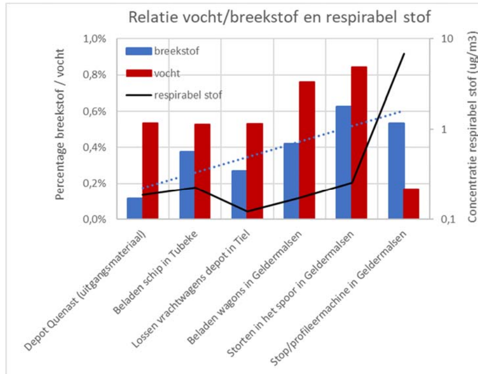
Afbeelding 25. Het vochtgehalte en percentage breekstof (<63µm) van de ballast gesteente na diverse handelingen en de concentratie respirabel stof, in µg/m 3 , gemeten tijdens deze handelingen.
