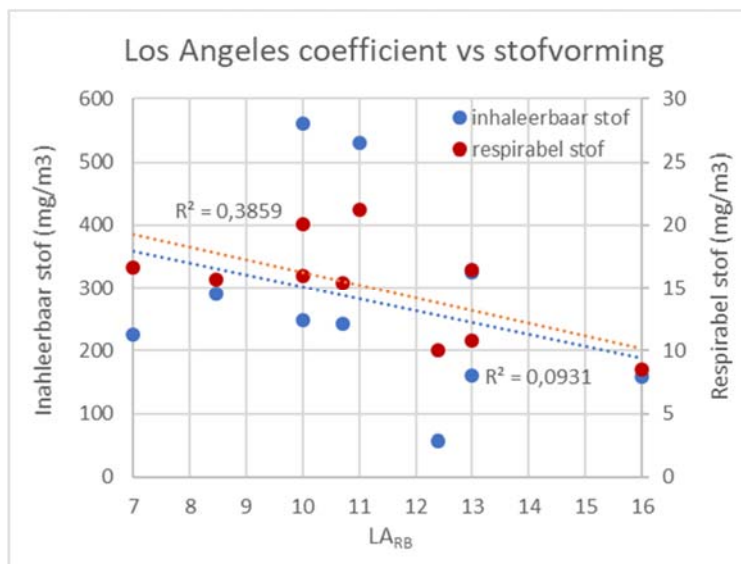
Afbeelding 19. Correlatiediagram van de inhaleerbaar- en respirabel stofconcentraties ( mg/m^3 ) gemeten tijdens de simulatie experimenten en de LA-waarde van de verschillende typen gesteenten.
