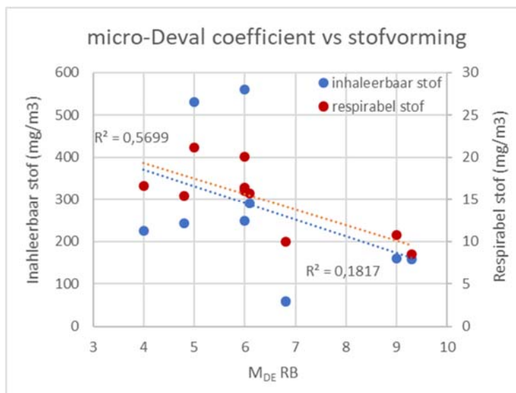
Afbeelding 20. Correlatiediagram van de inhaleerbaar- en respirabel stofconcentraties ( mg/m^3 ) gemeten tijdens de simulatie experimenten en de micro-Deval waarde van de verschillende typen gesteenten.
