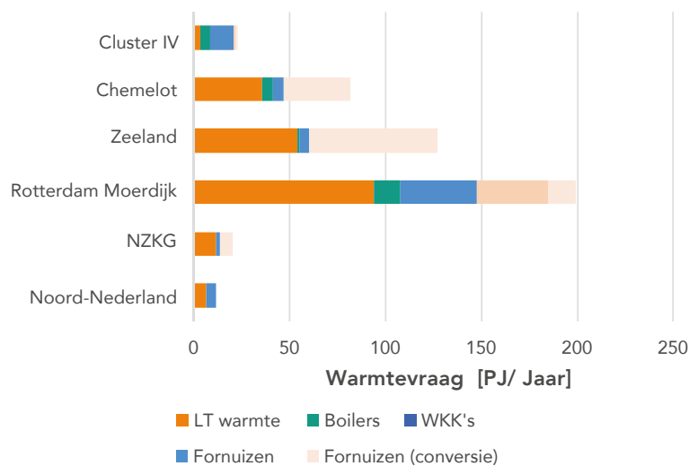
Figuur 2.3: Inschatting verdeling van LT en HT warmtegebruik in de Nederlandse industrie in 2018 naar sector en naar locatie.
