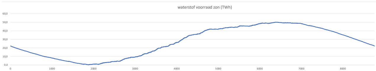
Figuur B2.12: Jaarverloop van waterstofvoorraad voor zon in directe elektrificatie.
