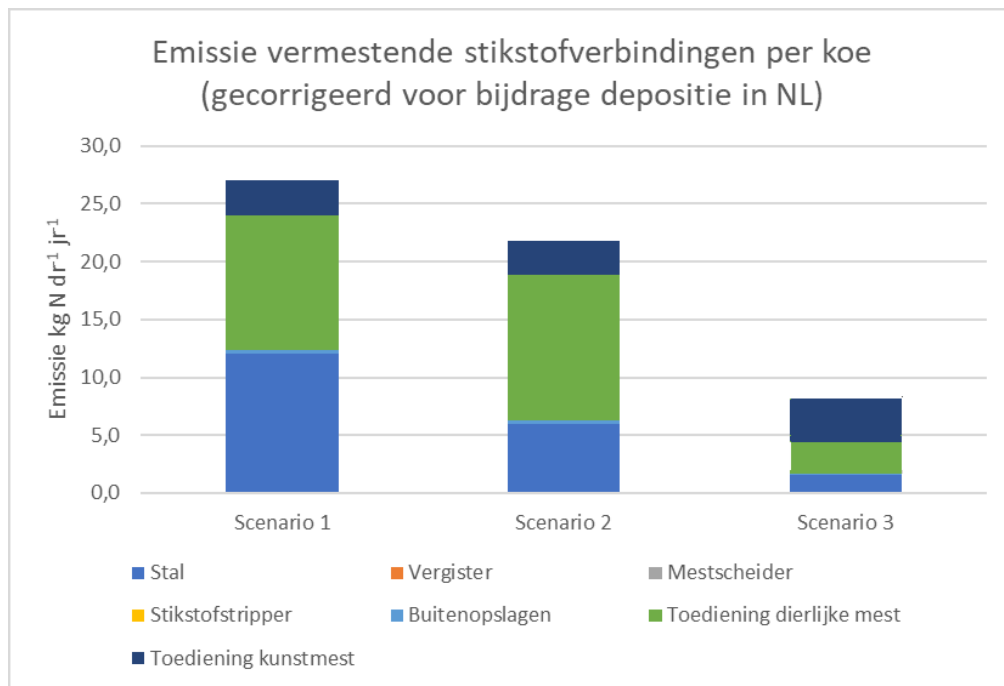
Figuur 1: Totaal van vermestende stikstofemissies ( \text{NH}_3 , \text{N}_2\text{O} en \text{NO} ) per bedrijfsonderdeel.
