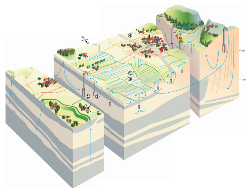
Figuur 1 3D-visualisatie van ondergrond, grondwaterstromen en land- en watergebruik rond Apeldoorn, gezien vanuit het noorden. (bron: Deltares/TNO, 2009).
