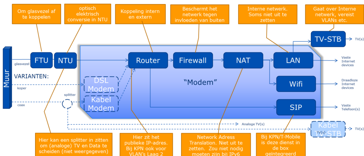
Figuur 1: Voorbeeld horizontale indeling netwerkaansluiting (glasvezel)
