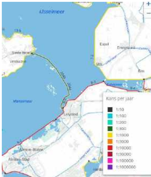
Figuur 5-1 Houtribdijk (204a en b) normen (ondergrens).
