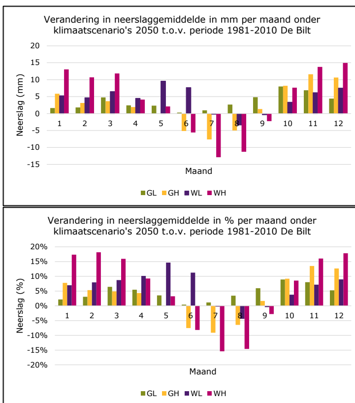
Figuur 7.1.4 Verandering van de neerslaggemiddelden in mm (boven) en procentueel (onder), per klimaatscenario per maand, ten opzichte van de neerslag in de periode 1981-2010 Data: KNMI 2014, figuur: eigen bewerking.
