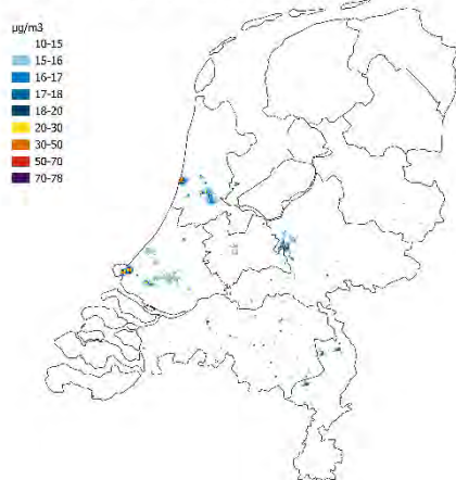
Jaargemiddelde PM 10 concentratie 2030 (VES)
