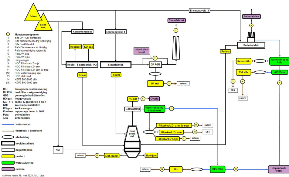
Figuur 4 Schematisch overzicht van de productie van ruwijzer uit erts en steenkool (Lips and Vooijs 2022)
