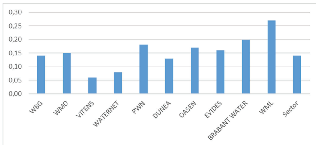
Prestatievergelijking 2019 Figuur 4.2 Elektriciteitsgebruik distributieproces 2019 per m3 distributie-input (kWh/m³)
