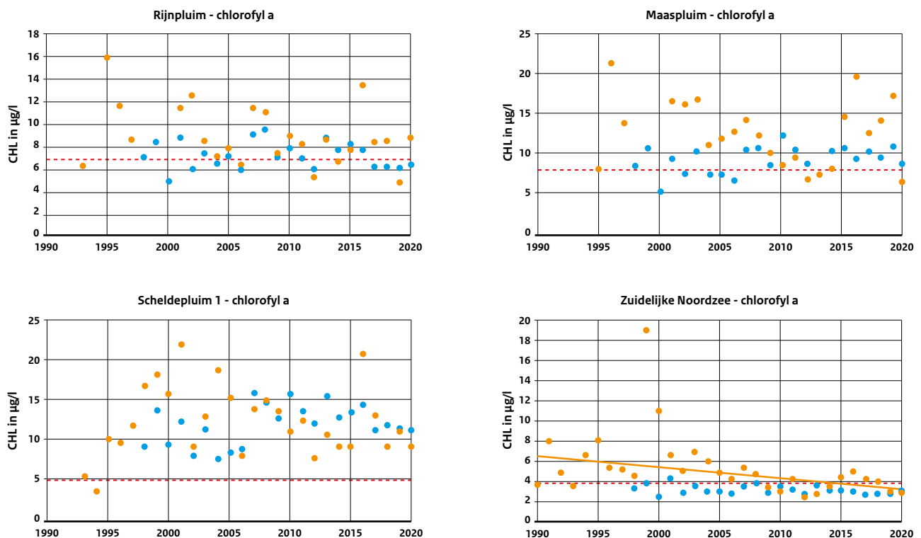
Figuur 5.7. Trend in groeiseizoen chlorofyl-a-concentraties in de rivierpluimen en de Zuidelijke Noordzee. Blauwe punten = satellietwaarnemingen; oranje punten = in-situ waarnemingen; onderbroken rode lijn = drempelwaarde; oranje getrokken lijn = trend (Sen's slope -2 procent per jaar). In de overige gebieden waar de Nederlandse Noordzee deel van uitmaakt zijn geen significante trends opgetreden.
