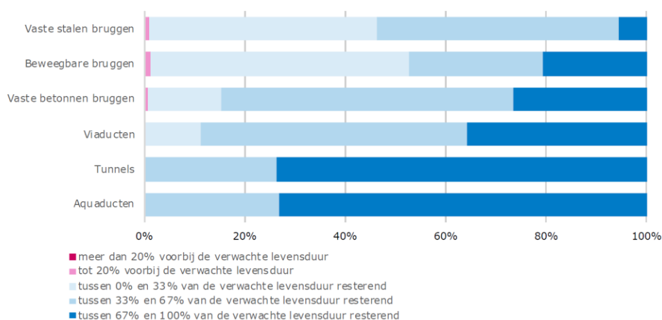
Figuur 10. Levensduur kunstwerken HWN als percentage van de totale verwachte levensduur (peildatum 1 januari 2020). 110
