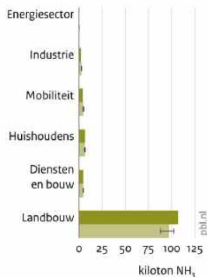
Ammoniak
