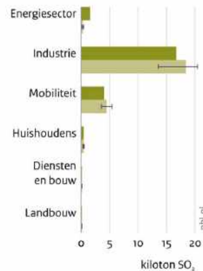
Zwaveldioxide
