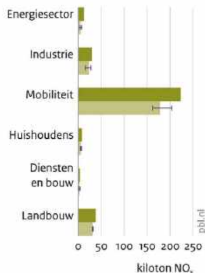
Stikstofoxiden
