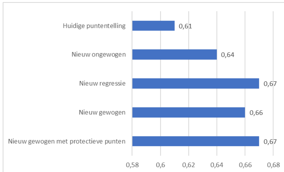
Figuur 9. AUC-waarden totaalscore gebaseerd op verschillende puntentellingen
