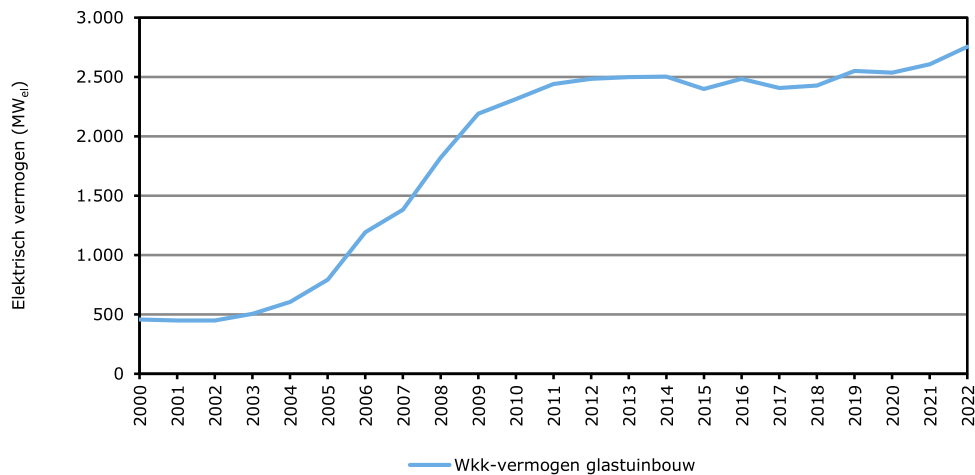
Figuur 4.1 Wkk-vermogen glastuinbouw v)
