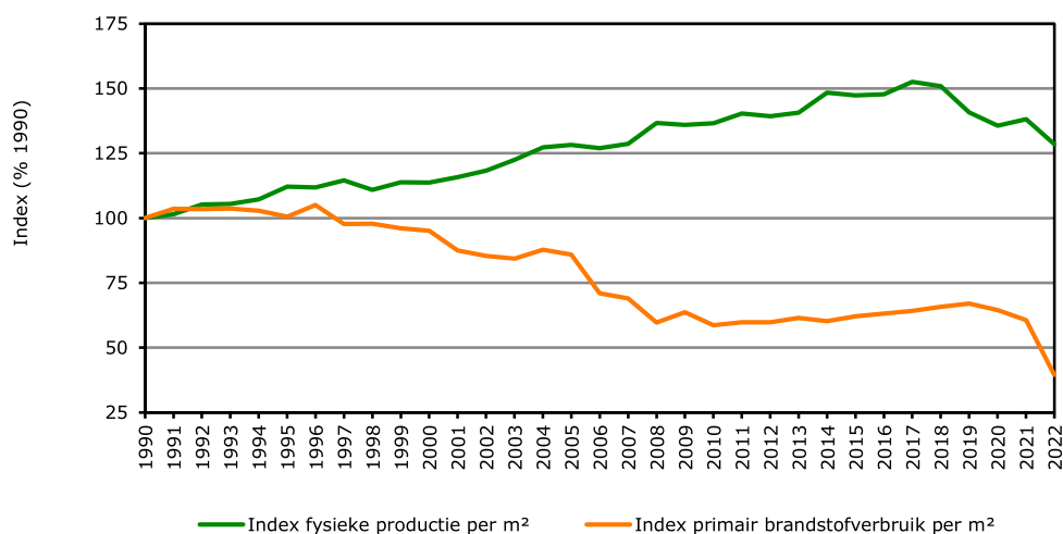
Figuur 2.8 Fysieke productie en primair brandstofverbruik in de productieglastuinbouw per m² kas v) v) Cijfers 2022 voorlopig
