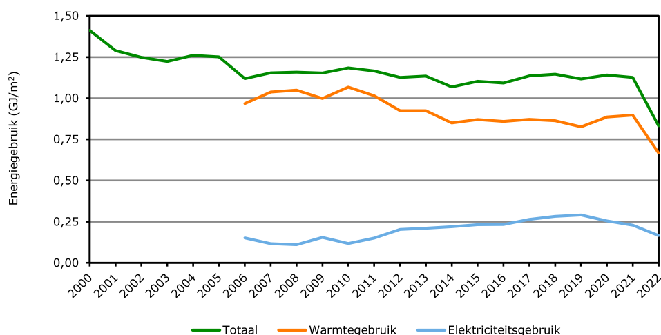
Figuur 2.6 Ontwikkeling gemiddeld energiegebruik glastuinbouw per m 2 na temperatuurcorrectie v) v) Cijfers 2022 voorlopig.
