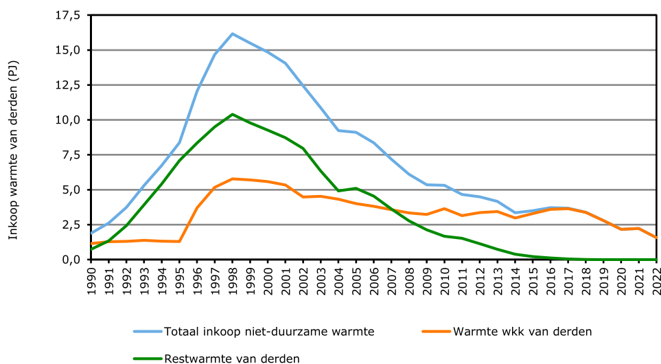
Figuur 4.6 Inkoop van niet-duurzame warmte van derden door de glastuinbouw v) v) Cijfers 2022 voorlopig.
