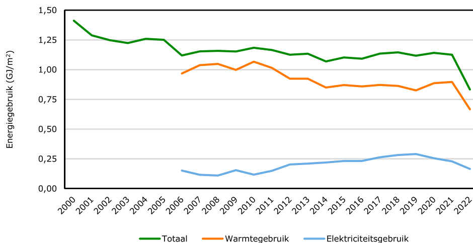
Figuur S.1 Ontwikkeling gemiddeld energiegebruik glastuinbouw per m 2 na temperatuurcorrectie v) v) Cijfers 2022 voorlopig.
