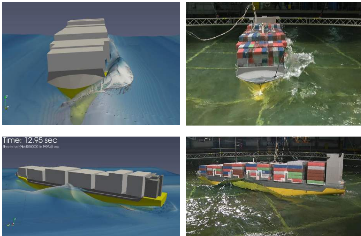
Vergelijk tussen COMFLOW CFD berekeningen en modelproeven in dwarsgolven (boven) en schuin-achterinkomende golven (onder)
