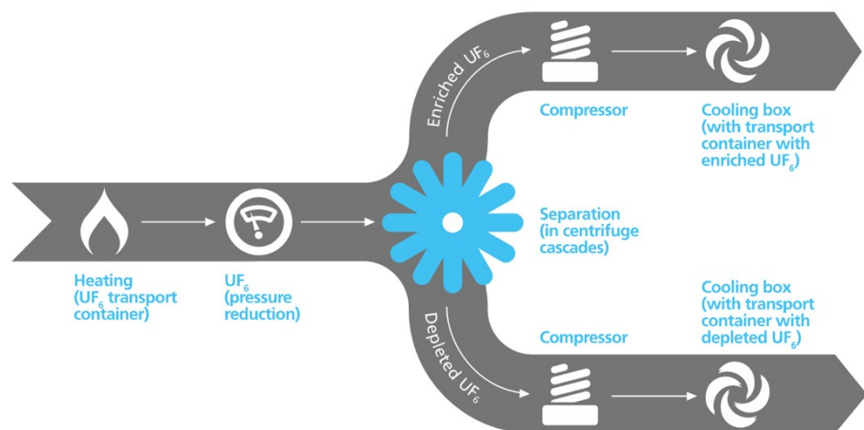
Figuur 1 Uraniumverrijkingsproces via ultracentrifuge, bron: Urenco.com
