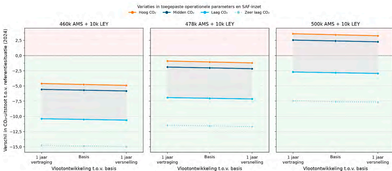
Figuur 15: Gecombineerd effect van variaties in verkeersvolume, operationele maatregelen, SAF-inzet en vlootontwikkeling (vlootvernieuwing en -verzwaring) op netto CO 2 -uitstoot van vluchten vertrekkend vanaf Schiphol en Lelystad Airport
