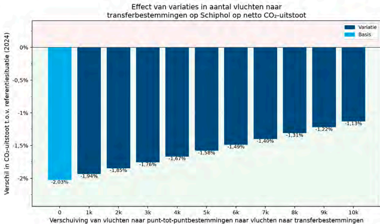
Figuur 6: Effect van variaties in het aantal extra vluchten van Schiphol naar transferbestemmingen op netto CO 2 -uitstoot van vluchten vertrekkend vanaf Schiphol en Lelystad Airport
