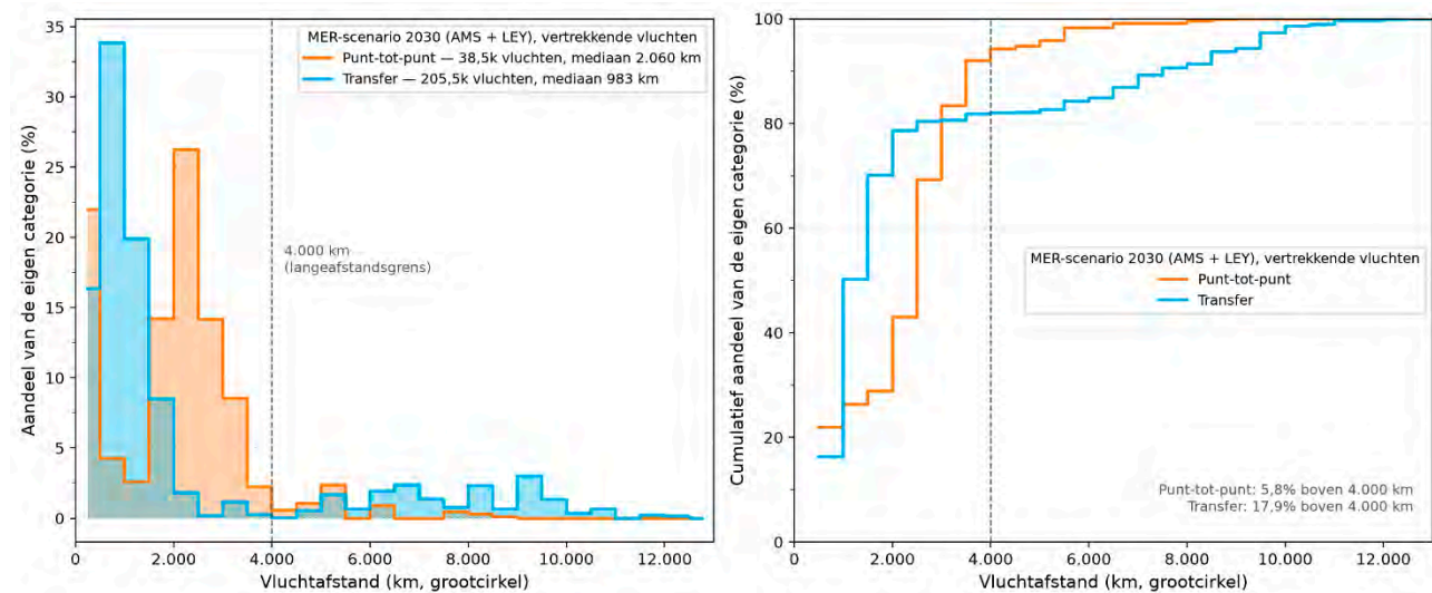
Figuur 5: Verdeling van punt-tot-punt- en transfervluchten over verschillende afstandsklassen in het mer- scenario
