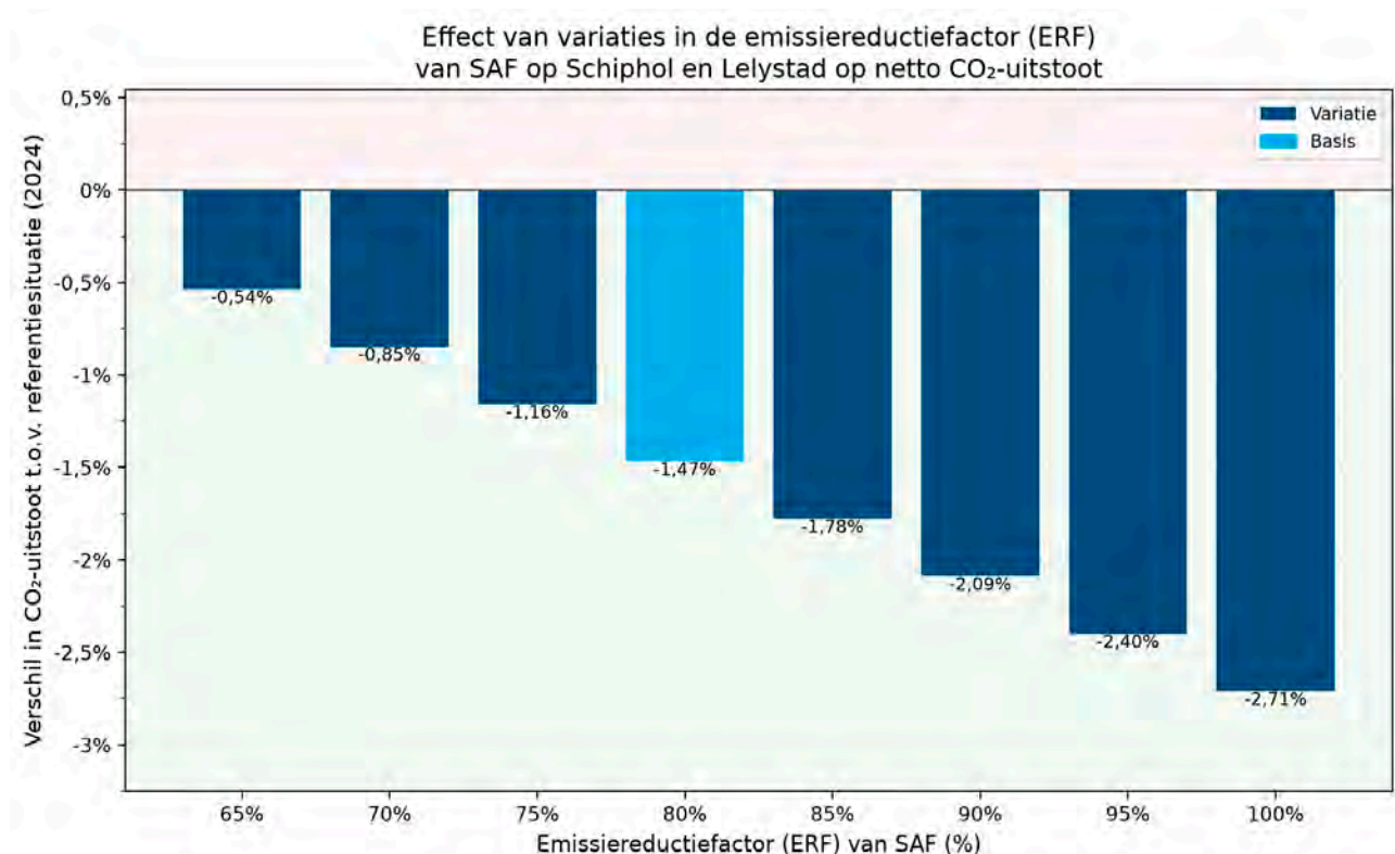
Figuur 28: Effect van variaties in de emissiereductiefactor (ERF) van SAF op netto CO 2 -uitstoot, berekend volgens alternatieve rekenmethodologie
