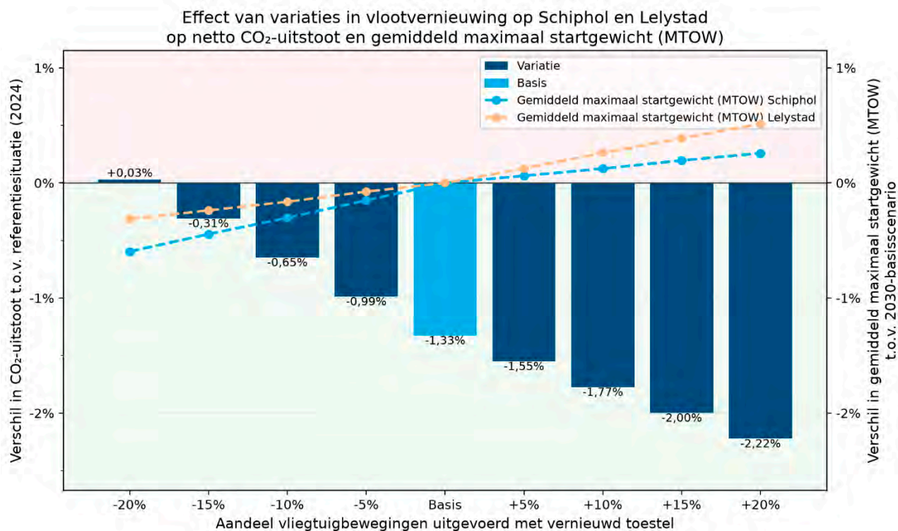
Figuur 20: Effect van variaties in vlootvernieuwing op netto CO 2 -uitstoot en gemiddeld maximaal startgewicht (MTOW) van vluchten vertrekkend vanaf Schiphol en Lelystad Airport (ten opzichte van referentiesituatie op basis van gebruiksjaar 2024)
