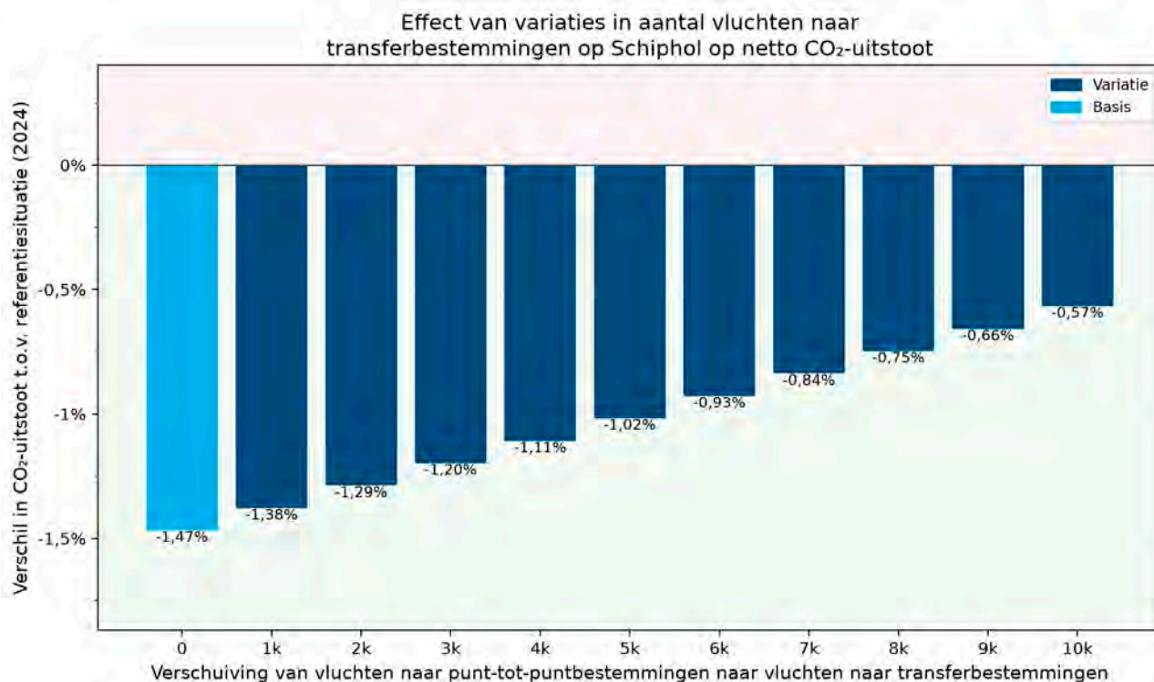
Figuur 30: Effect van variaties in het aantal extra vluchten van Schiphol naar transferbestemmingen op netto CO 2 -uitstoot van vluchten vertrekkend vanaf Schiphol en Lelystad Airport (met CORSIA-berekeningsmethode voor effecten van SAF)
