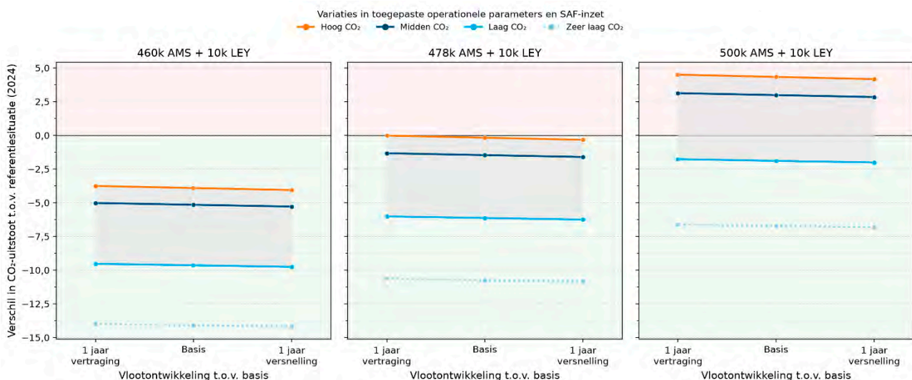
Figuur 38: Gecombineerd effect van variaties in verkeersvolume, operationele maatregelen, SAF-inzet en vlootontwikkeling (vlootvernieuwing en -verzwaring) op netto CO 2 -uitstoot van vluchten vertrekkend vanaf Schiphol en Lelystad Airport (met CORSIA-berekeningsmethode voor effecten van SAF)
