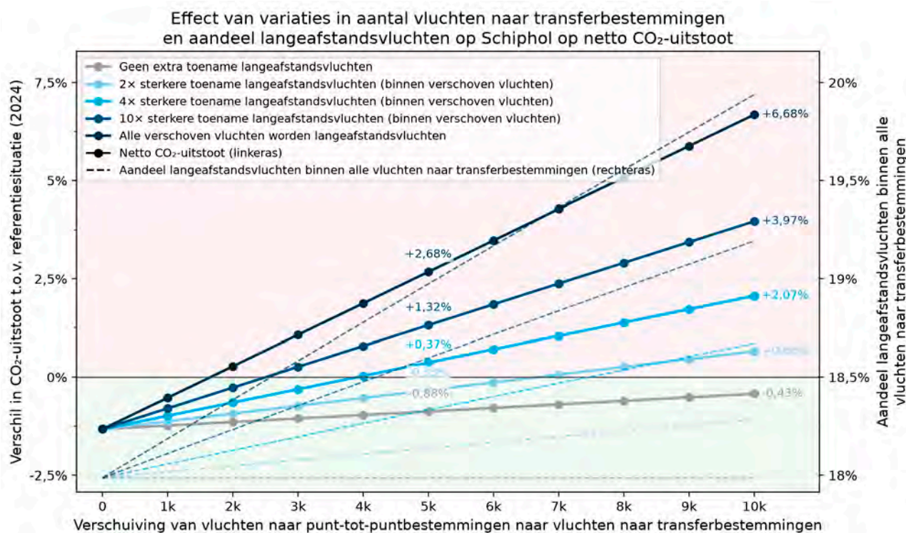
Figuur 19: Effect van variaties in extra vluchten van Schiphol naar transferbestemmingen verder dan 4.000 kilometer op netto CO 2 -uitstoot van vluchten vertrekkend vanaf Schiphol en Lelystad Airport (ten opzichte van referentiesituatie op basis van gebruiksjaar 2024)
