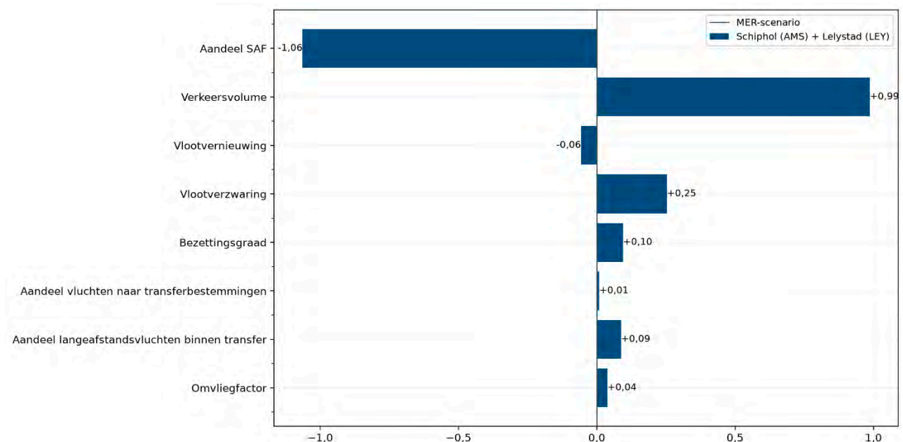
Figuur 1: Het lineaire effect van 1 procentpunt-verandering van elke parameter op de gemiddelde netto CO 2 -uitstoot van vluchten vanaf Schiphol en Lelystad Airport
