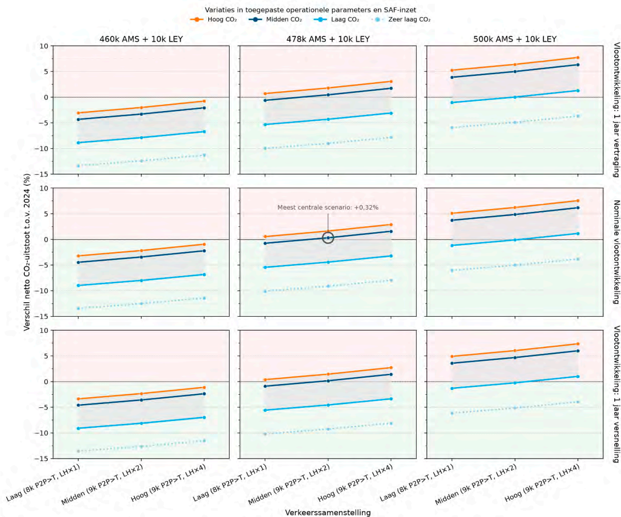
Figuur 39: Gecombineerd effect van variaties in verkeersvolume, operationele maatregelen, SAF-inzet, vlootontwikkeling (vlootvernieuwing en -verzwaring) en verkeerssamenstelling op netto CO 2 -uitstoot (met CORSIA-berekeningsmethode voor effecten van SAF)
