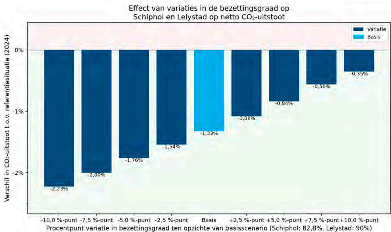
Figuur 23: Effect van variaties in de bezettingsgraad op netto CO 2 -uitstoot van vluchten vertrekkend vanaf Schiphol en Lelystad Airport (ten opzichte van referentiesituatie op basis van gebruiksjaar 2024)
