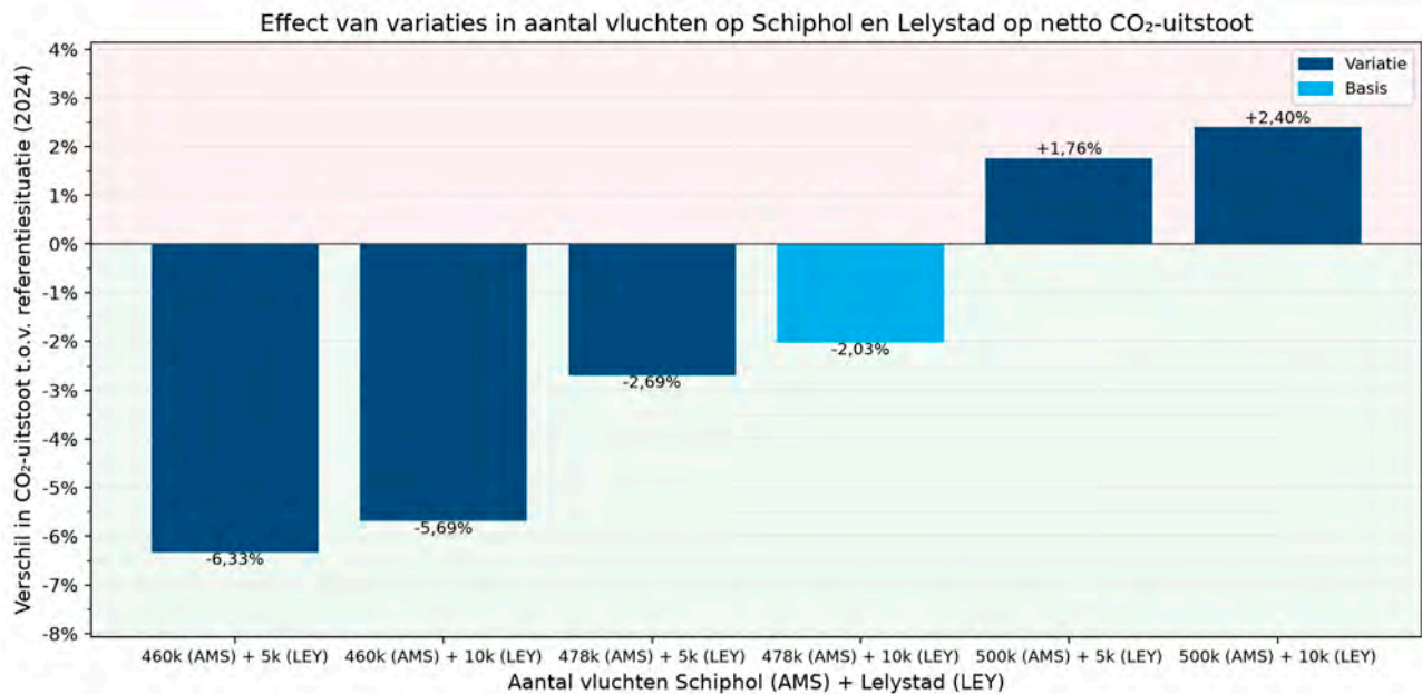
Figuur 4: Effect van variaties in verkeersvolume op netto CO 2 -uitstoot van vluchten vertrekkend vanaf Schiphol en Lelystad Airport
