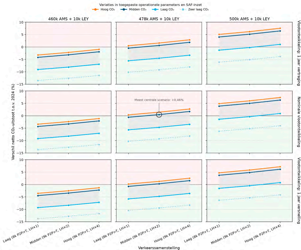
Figuur 27: Gecombineerd effect van variaties in verkeersvolume, operationele maatregelen, SAF-inzet, vlootontwikkeling (vlootvernieuwing en -verzwaring) en verkeerssamenstelling op netto CO 2 -uitstoot (ten opzichte van referentiesituatie op basis van gebruiksjaar 2024)
