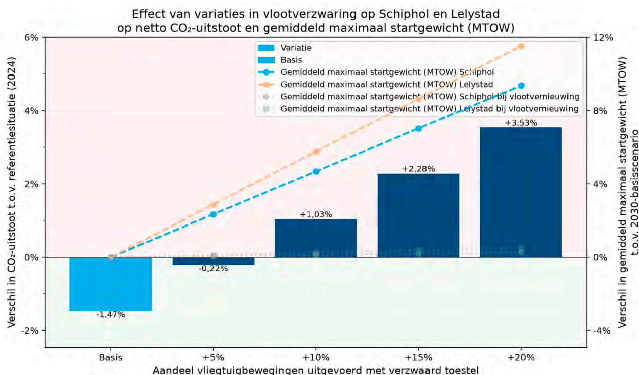
Figuur 33: Effect van variaties in vlootverzwaring op netto CO 2 -uitstoot en gemiddeld maximaal startgewicht (MTOW) van vluchten vertrekkend vanaf Schiphol en Lelystad Airport (met CORSIA-berekeningsmethode voor effecten van SAF)
