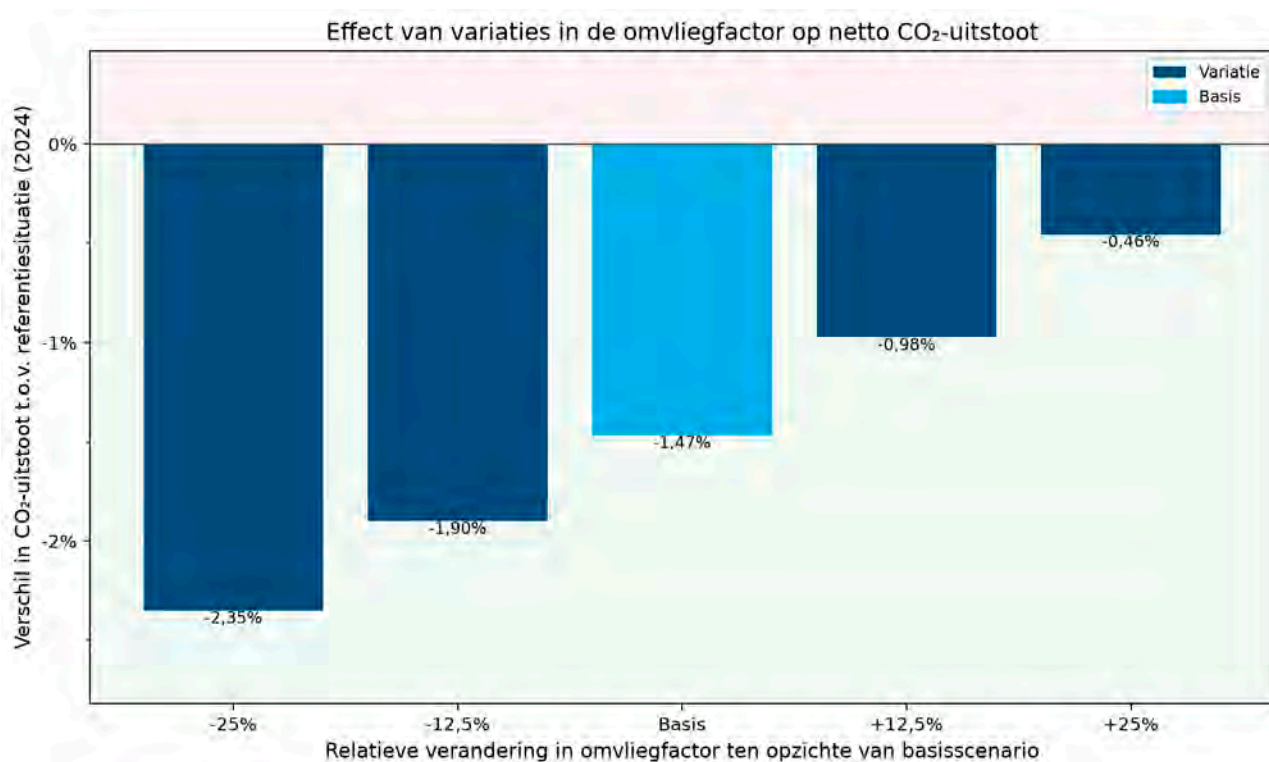
Figuur 36: Effect van variaties in de omvliegfactor op netto CO 2 -uitstoot van vluchten vertrekkend vanaf Schiphol en Lelystad Airport (met CORSIA-berekeningsmethode voor effecten van SAF)
