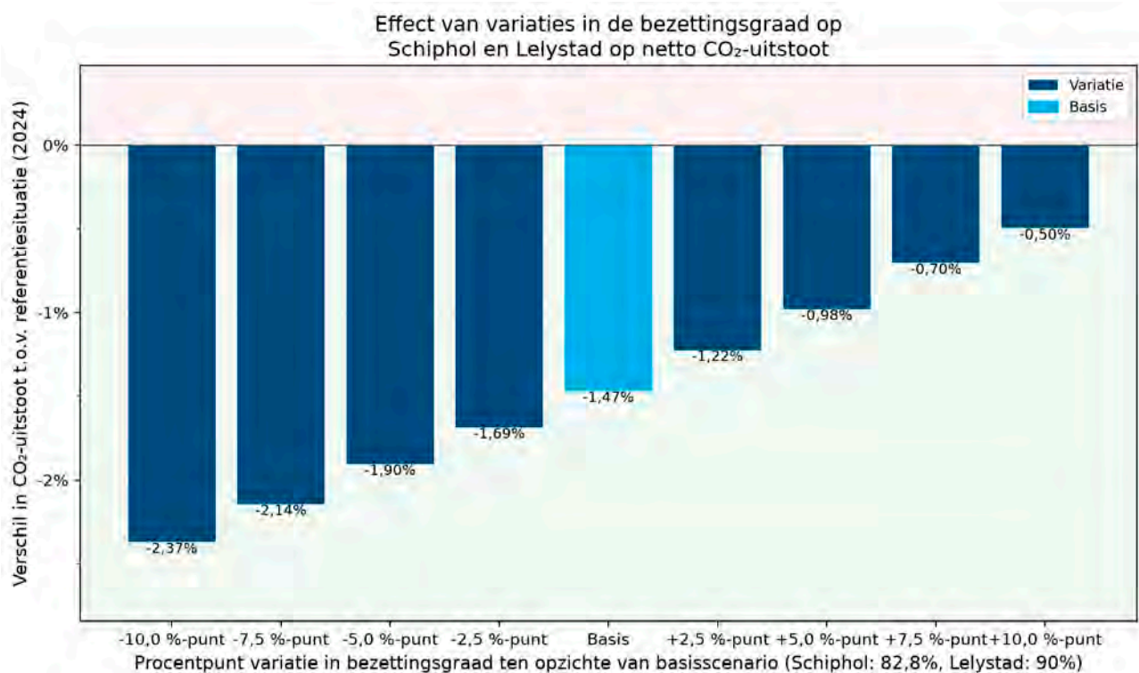
Figuur 35: Effect van variaties in de bezettingsgraad op netto CO 2 -uitstoot van vluchten vertrekkend vanaf Schiphol en Lelystad Airport (met CORSIA-berekeningsmethode voor effecten van SAF)
