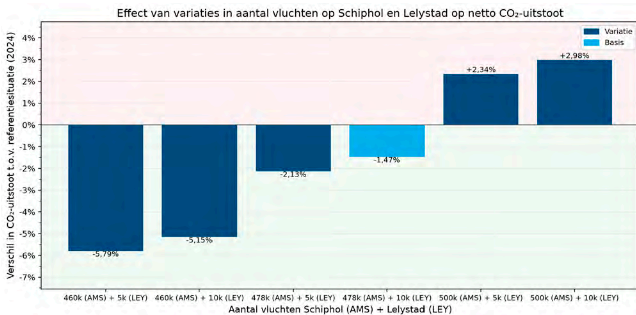
Figuur 29: Effect van variaties in verkeersvolume op netto CO 2 -uitstoot van vluchten vertrekkend vanaf Schiphol en Lelystad Airport (met CORSIA-berekeningsmethode voor effecten van SAF)
