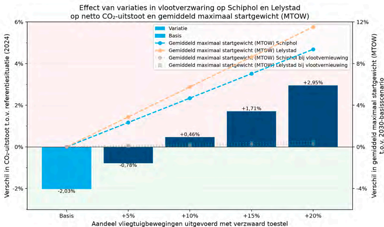
Figuur 9: Effect van variaties in vlootverzwaring op netto CO 2 -uitstoot en gemiddeld maximaal startgewicht (MTOW) van vluchten vertrekkend vanaf Schiphol en Lelystad Airport
