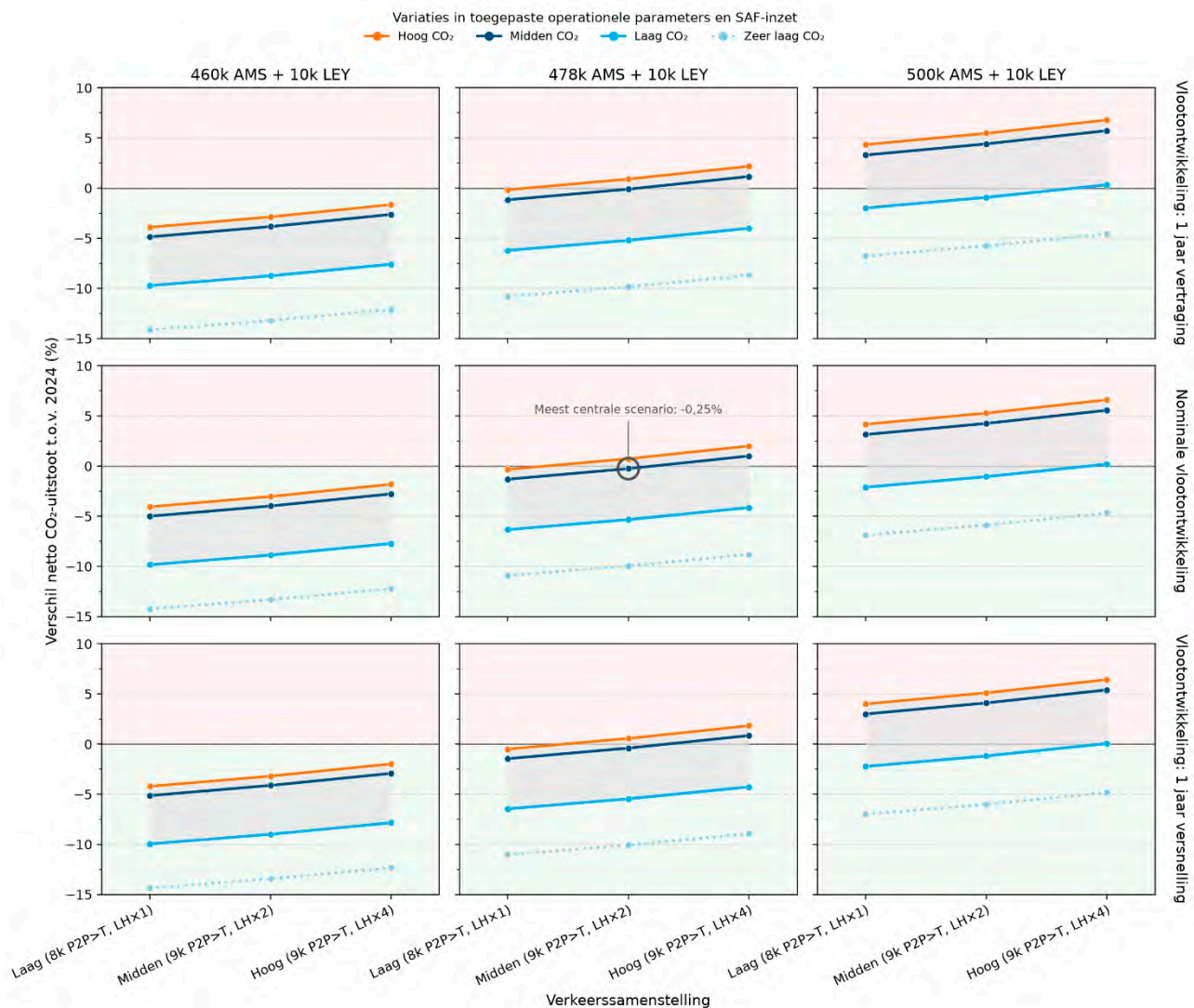
Figuur 16: Gecombineerd effect van variaties in verkeersvolume, operationele maatregelen, SAF-inzet, vlootontwikkeling (vlootvernieuwing en -verzwaring) en verkeerssamenstelling op netto CO 2 -uitstoot van vluchten vertrekkend vanaf Schiphol en Lelystad Airport (bij de verkeerssamenstelling duidt P2P>T een verschuiving van punt-tot-punt- naar transfervluchten aan en LHx een eventuele sterkere toename in langeafstandsvluchten)
