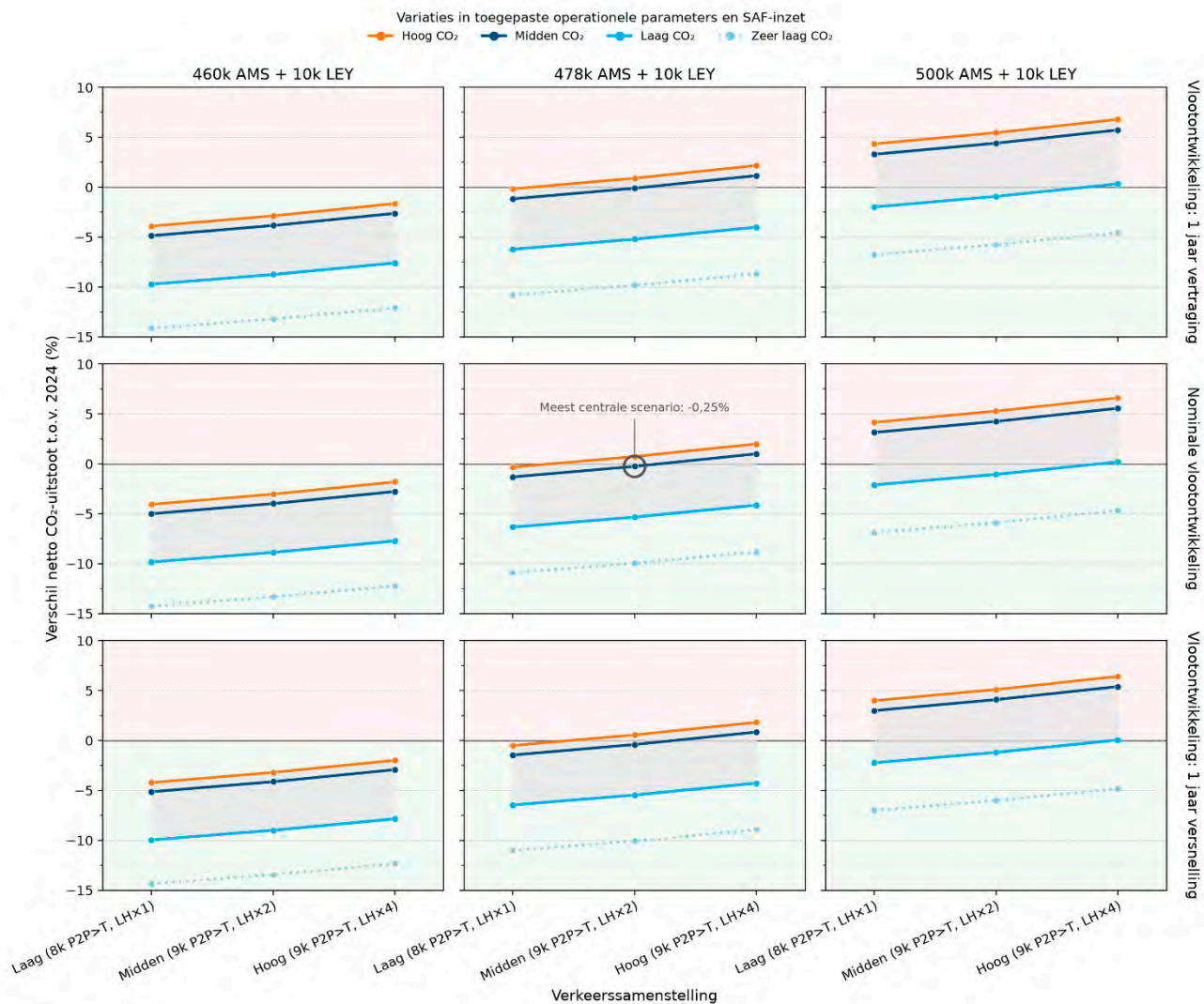
Figuur 2: Gecombineerd effect van variaties in verkeersvolume, operationele maatregelen, SAF-inzet, vlootontwikkeling (vlootvernieuwing en -verzwaring) en verkeerssamenstelling op netto CO 2 -uitstoot van vluchten vertrekkend vanaf Schiphol en Lelystad Airport (bij de verkeerssamenstelling duidt P2P>T een verschuiving van punt-tot-punt- naar transfervluchten aan en LH× een eventuele sterkere toename in langeafstandsvluchten)
