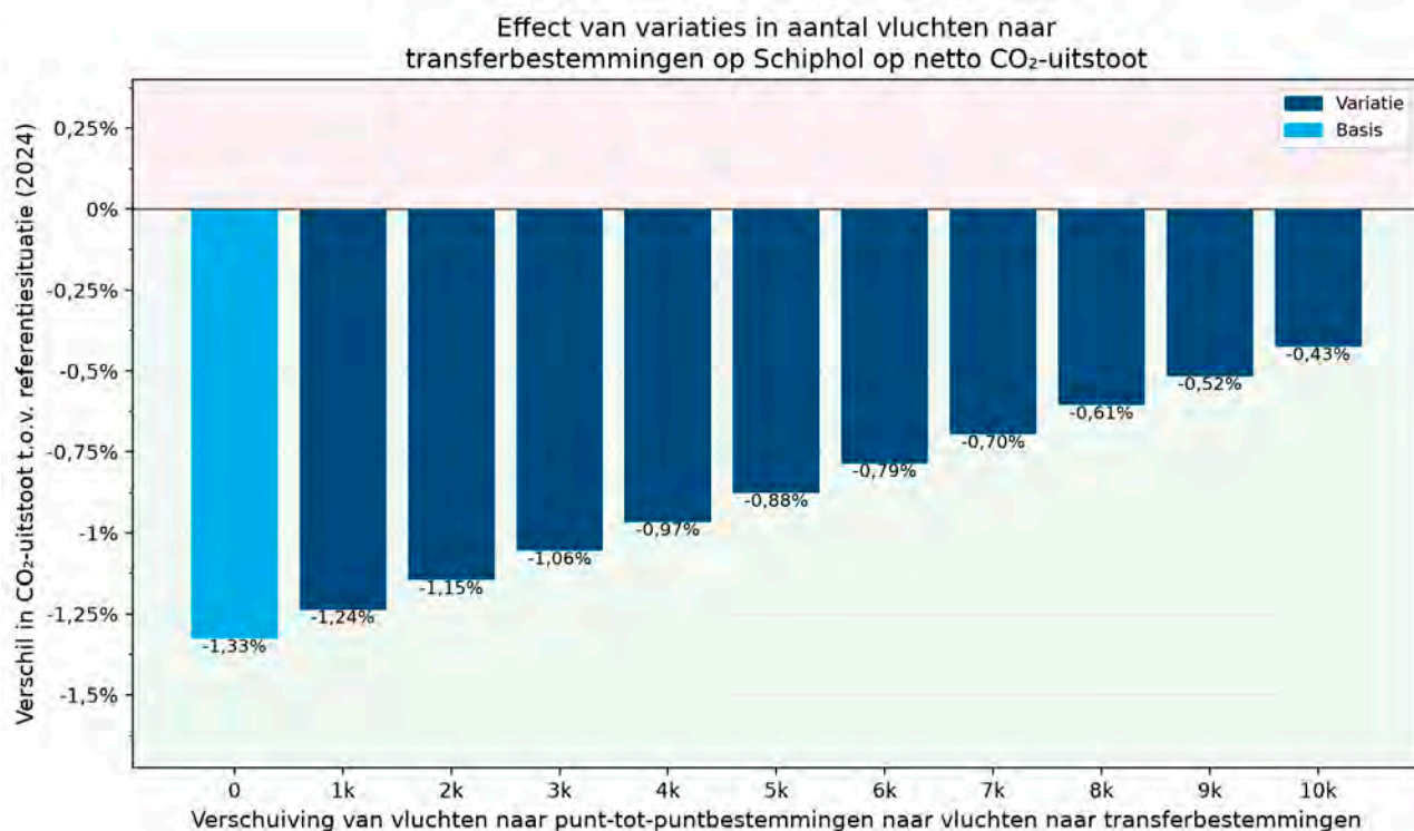
Figuur 18: Effect van variaties in het aantal extra vluchten van Schiphol naar transferbestemmingen op netto CO 2 -uitstoot van vluchten vertrekkend vanaf Schiphol en Lelystad Airport (ten opzichte van referentiesituatie op basis van gebruiksjaar 2024)
