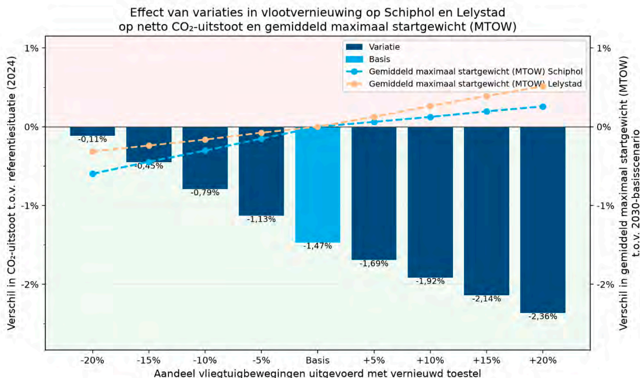
Figuur 32: Effect van variaties in vlootvernieuwing op netto CO 2 -uitstoot en gemiddeld maximaal startgewicht (MTOW) van vluchten vertrekkend vanaf Schiphol en Lelystad Airport (met CORSIA-berekeningsmethode voor effecten van SAF)
