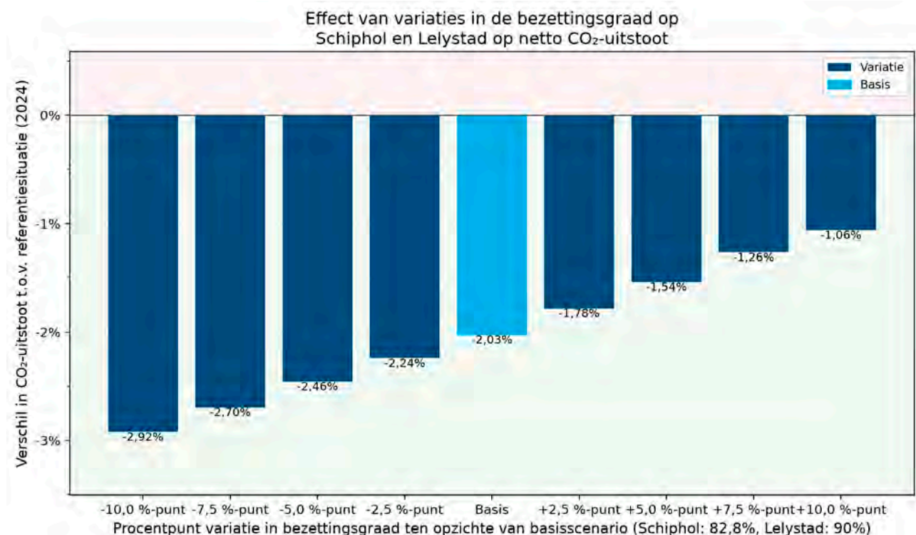
Figuur 11: Effect van variaties in de bezettingsgraad op netto CO 2 -uitstoot van vluchten vertrekkend vanaf Schiphol en Lelystad Airport
