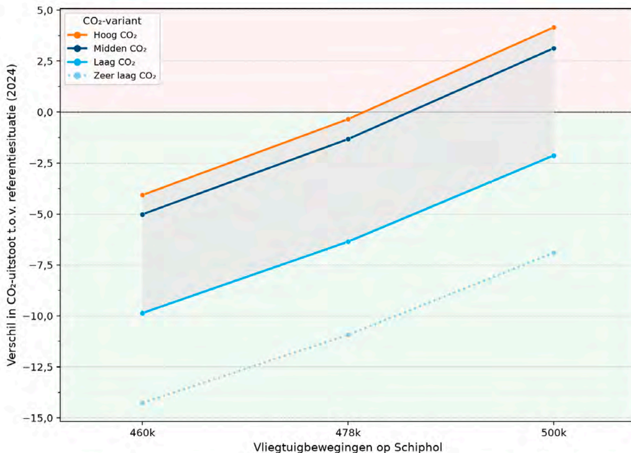
Figuur 25: Gecombineerd effect van variaties in verkeersvolume, operationele maatregelen en SAF-inzet op netto CO 2 -uitstoot van vluchten vertrekkend vanaf Schiphol en Lelystad Airport (ten opzichte van referentiesituatie op basis van gebruiksjaar 2024)
