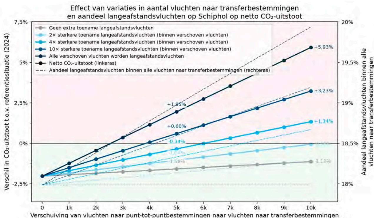
Figuur 7: Effect van variaties in extra vluchten van Schiphol naar transferbestemmingen verder dan 4.000 kilometer op netto CO 2 -uitstoot van vluchten vertrekkend vanaf Schiphol en Lelystad Airport
