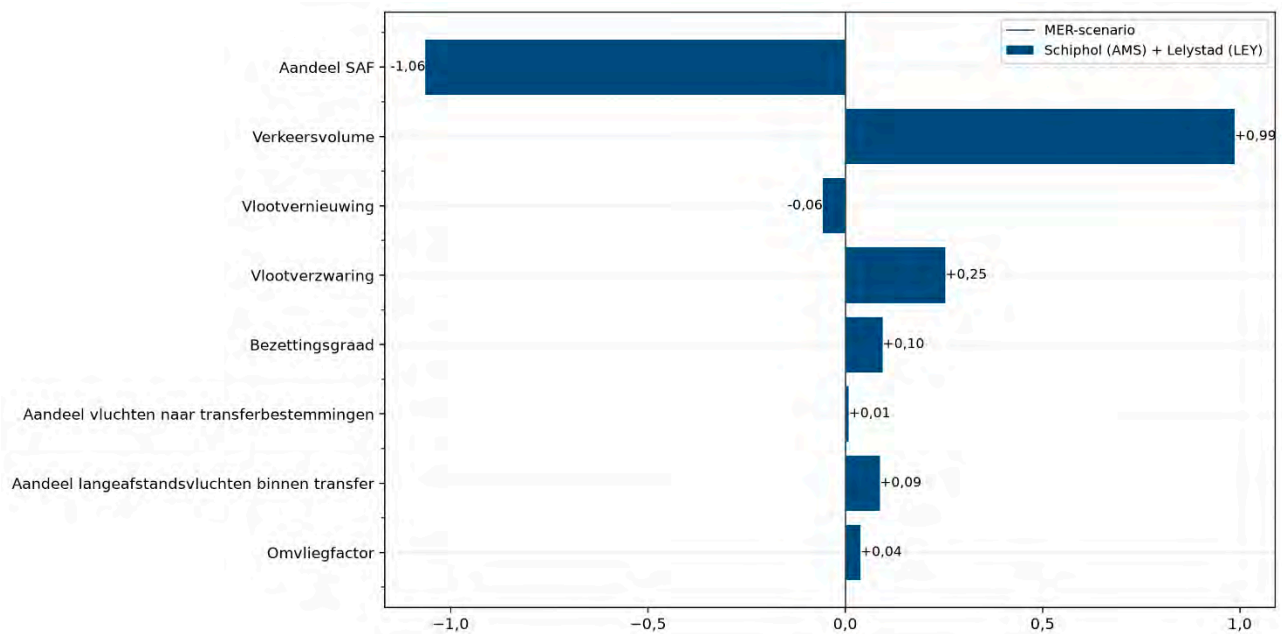
Figuur 13: Gemiddelde lineaire variatie in netto CO 2 -uitstoot van vluchten vertrekkend vanaf Schiphol en Lelystad Airport ten gevolge van een 1 procentpunt toename van elk van de onderzochte parameters
