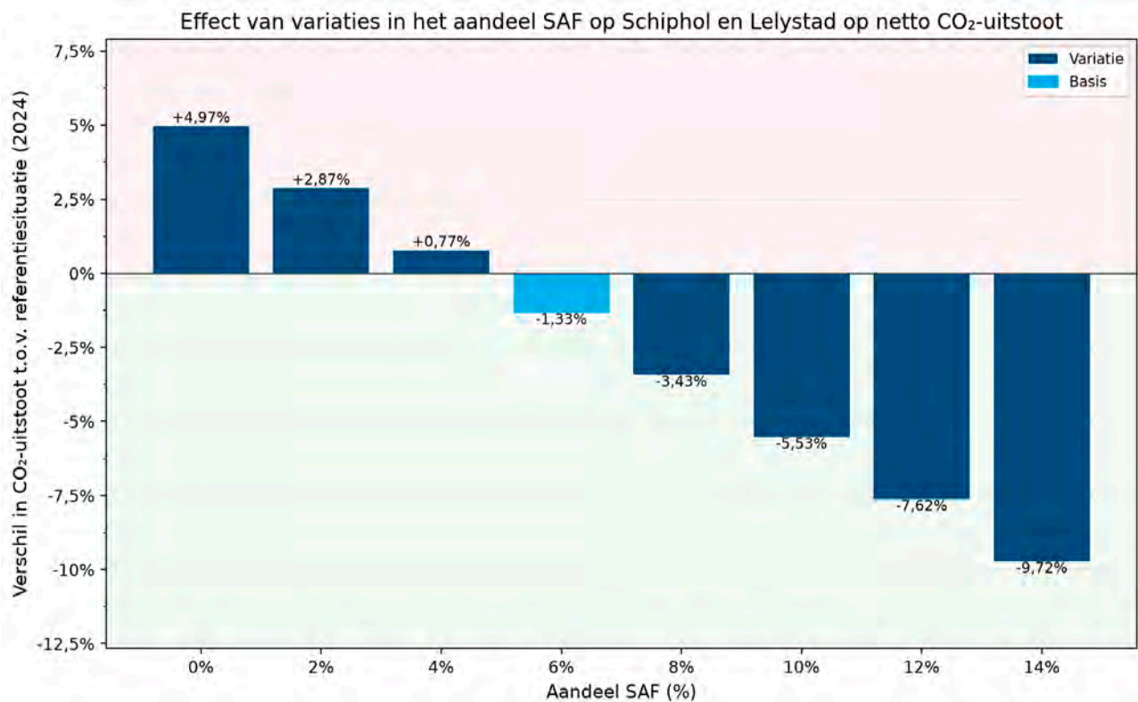
Figuur 22: Effect van variaties in het aandeel SAF op netto CO 2 -uitstoot van vluchten vertrekkend vanaf Schiphol en Lelystad Airport (ten opzichte van referentiesituatie op basis van gebruiksjaar 2024)
