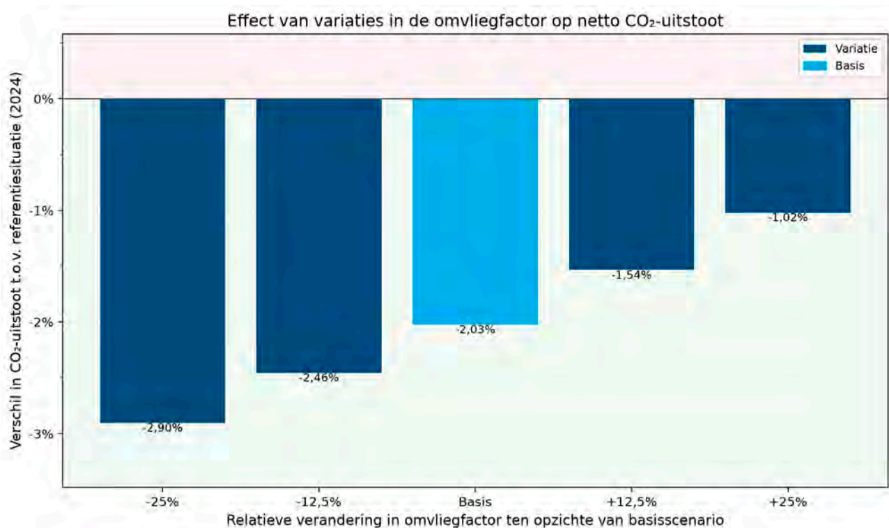
Figuur 12: Effect van variaties in de omvliegfactor op netto CO 2 -uitstoot van vluchten vertrekkend vanaf Schiphol en Lelystad Airport
