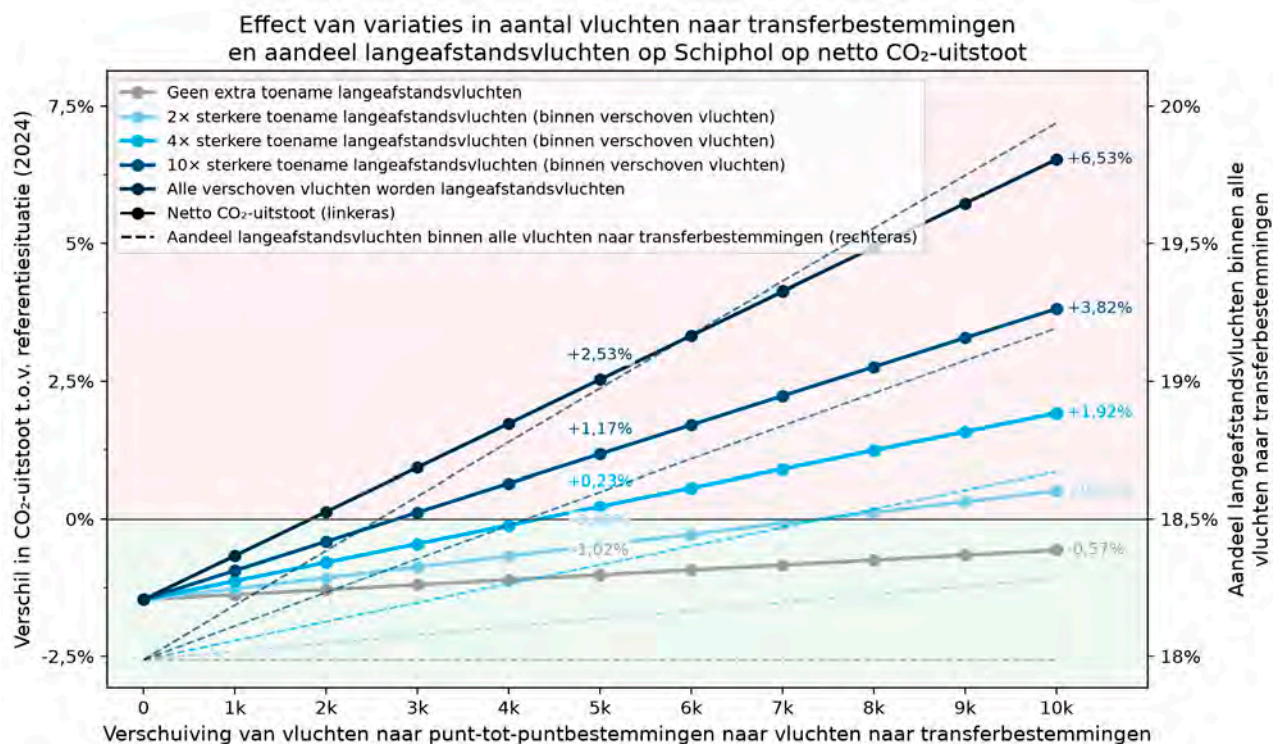
Figuur 31: Effect van variaties in extra vluchten van Schiphol naar transferbestemmingen verder dan 4.000 kilometer op netto CO 2 -uitstoot van vluchten vertrekkend vanaf Schiphol en Lelystad Airport (met CORSIA-berekeningsmethode voor effecten van SAF)
