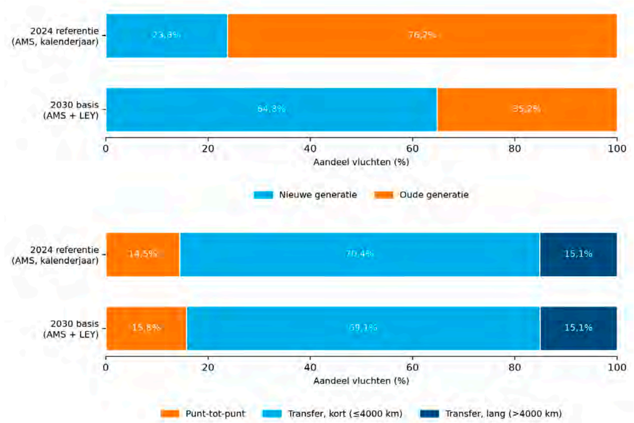
Figuur 3: Vloot- en netwerkeigenschappen (bestemmingen) van de referentiesituatie en het mer-scenario
