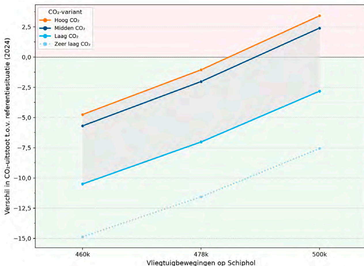
Figuur 14: Gecombineerd effect van variaties in verkeersvolume, operationele maatregelen en SAF-inzet op netto CO 2 -uitstoot van vluchten vertrekkend vanaf Schiphol en Lelystad Airport
