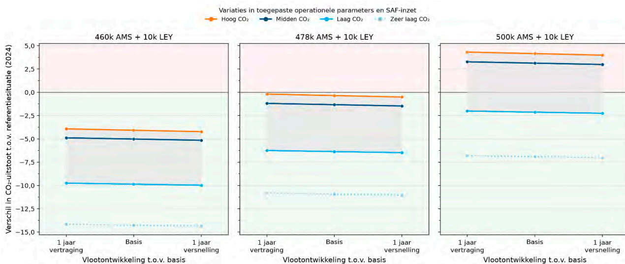
Figuur 26: Gecombineerd effect van variaties in verkeersvolume, operationele maatregelen, SAF-inzet en vlootontwikkeling (vlootvernieuwing en -verzwaring) op netto CO 2 -uitstoot van vluchten vertrekkend vanaf Schiphol en Lelystad Airport (ten opzichte van referentiesituatie op basis van gebruiksjaar 2024)
