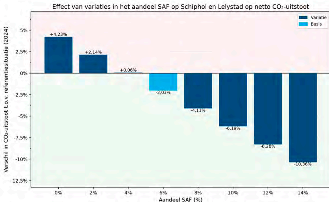
Figuur 10: Effect van variaties in het aandeel SAF op netto CO 2 -uitstoot van vluchten vertrekkend vanaf Schiphol en Lelystad Airport
