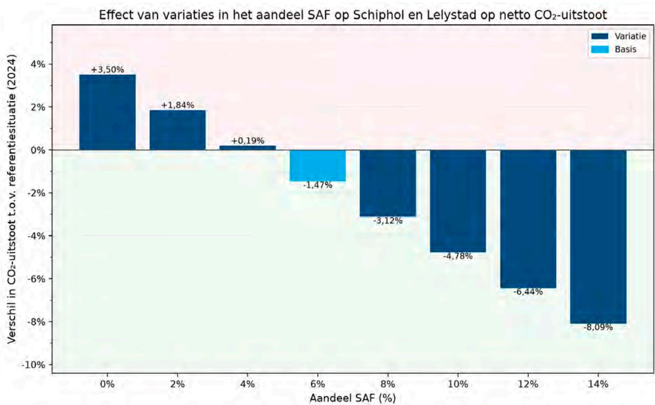
Figuur 34: Effect van variaties in het aandeel SAF op netto CO 2 -uitstoot van vluchten vertrekkend vanaf Schiphol en Lelystad Airport (met CORSIA-berekeningsmethode voor effecten van SAF)
