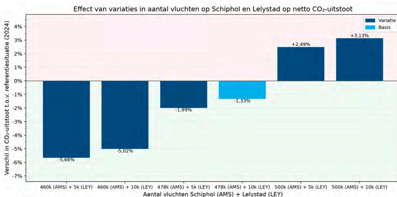
Figuur 17: Effect van variaties in verkeersvolume op netto CO 2 -uitstoot van vluchten vertrekkend vanaf Schiphol en Lelystad Airport (ten opzichte van referentiesituatie op basis van gebruiksjaar 2024)
