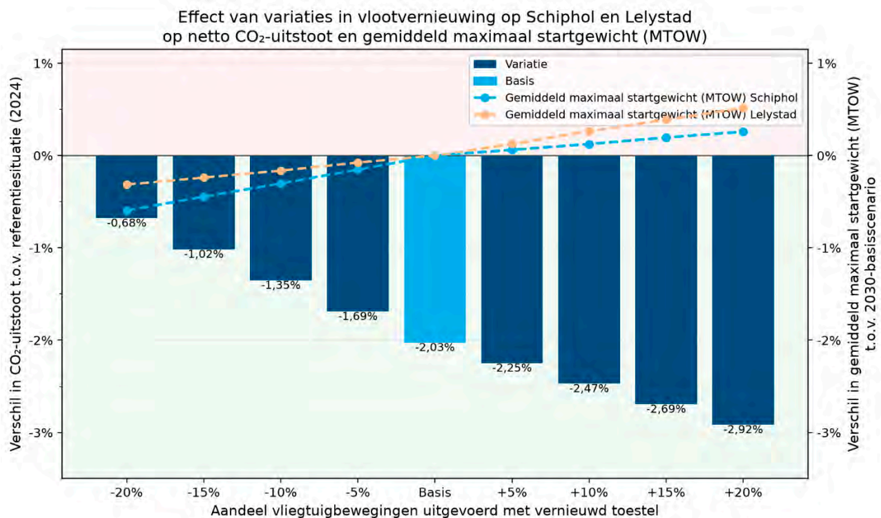
Figuur 8: Effect van variaties in vlootvernieuwing op netto CO 2 -uitstoot en gemiddeld maximaal startgewicht (MTOW) van vluchten vertrekkend vanaf Schiphol en Lelystad Airport
