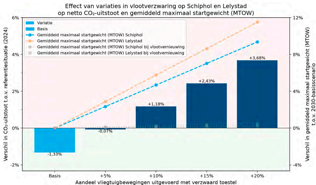
Figuur 21: Effect van variaties in vlootverzwaring op netto CO 2 -uitstoot en gemiddeld maximaal startgewicht (MTOW) van vluchten vertrekkend vanaf Schiphol en Lelystad Airport (ten opzichte van referentiesituatie op basis van gebruiksjaar 2024)
