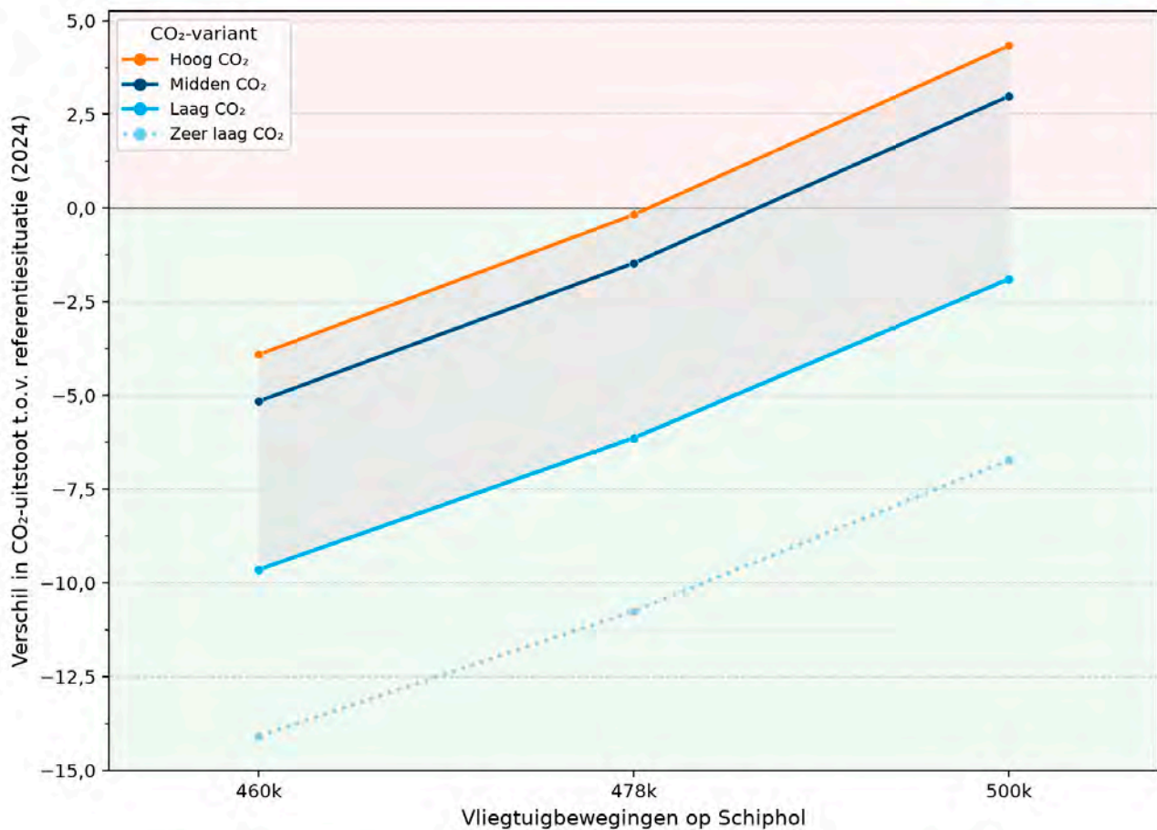
Figuur 37: Gecombineerd effect van variaties in verkeersvolume, operationele maatregelen en SAF-inzet op netto CO 2 -uitstoot van vluchten vertrekkend vanaf Schiphol en Lelystad Airport (met CORSIA-berekeningsmethode voor effecten van SAF)
