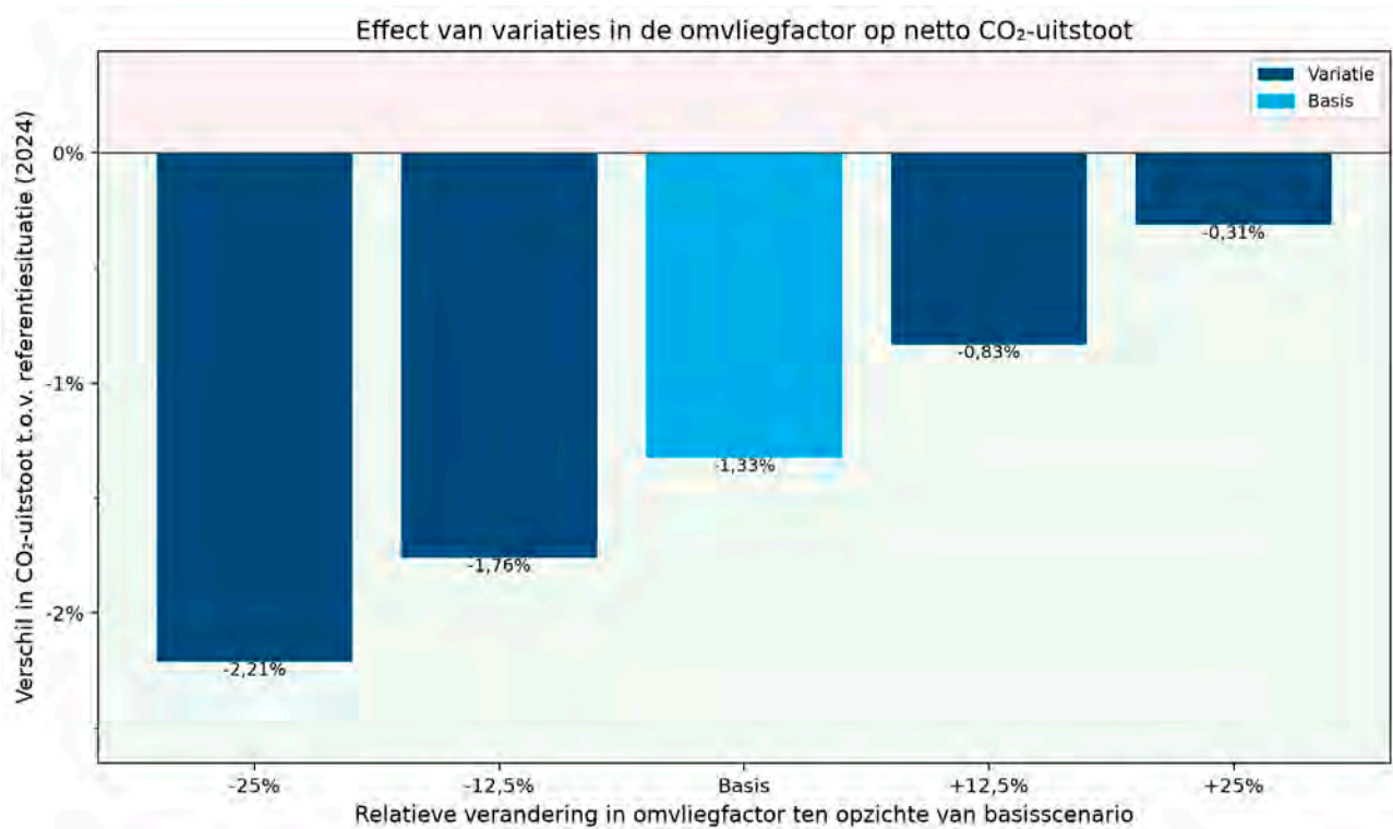
Figuur 24: Effect van variaties in de omvliegfactor op netto CO 2 -uitstoot van vluchten vertrekkend vanaf Schiphol en Lelystad Airport (ten opzichte van referentiesituatie op basis van gebruiksjaar 2024)
